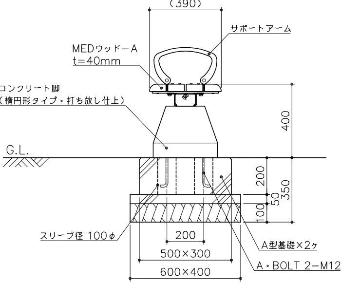
側面図 S= 1 : 20
