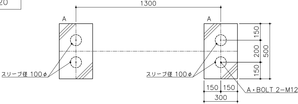
立面図 S= 1 : 20
