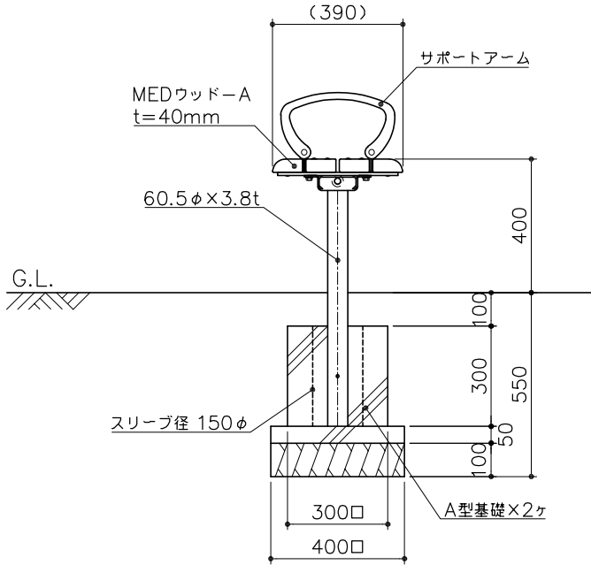
側面図 S= 1 : 20
