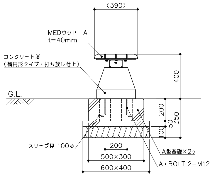
側面図 S= 1:20
