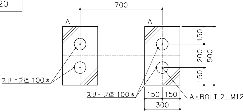
立面図 S= 1 : 20
