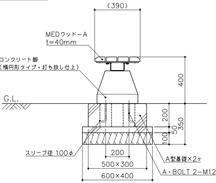
側面図 S= 1 : 20
