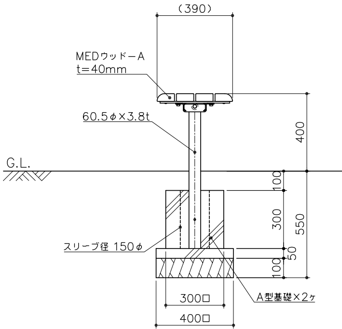
側面図 S= 1 : 20
