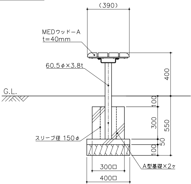
側面図 S= 1 : 20
