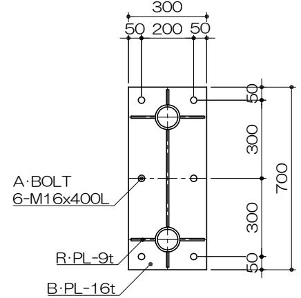
アンカープラン S= 1 : 20
