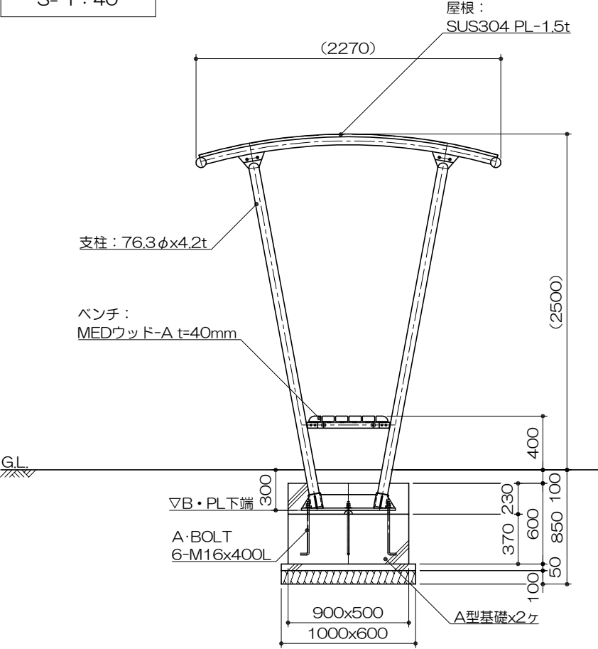
側面図 S= 1 : 40
