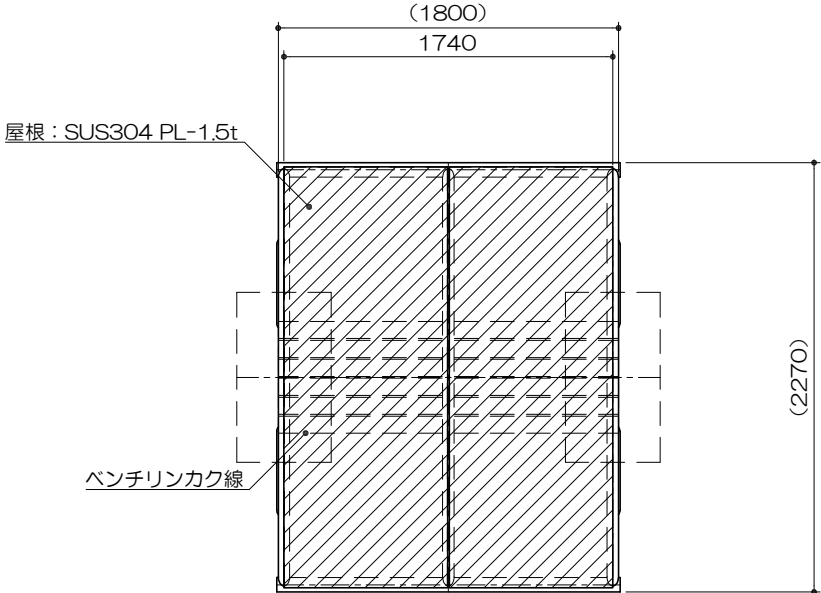
平面図 S= 1 : 40
