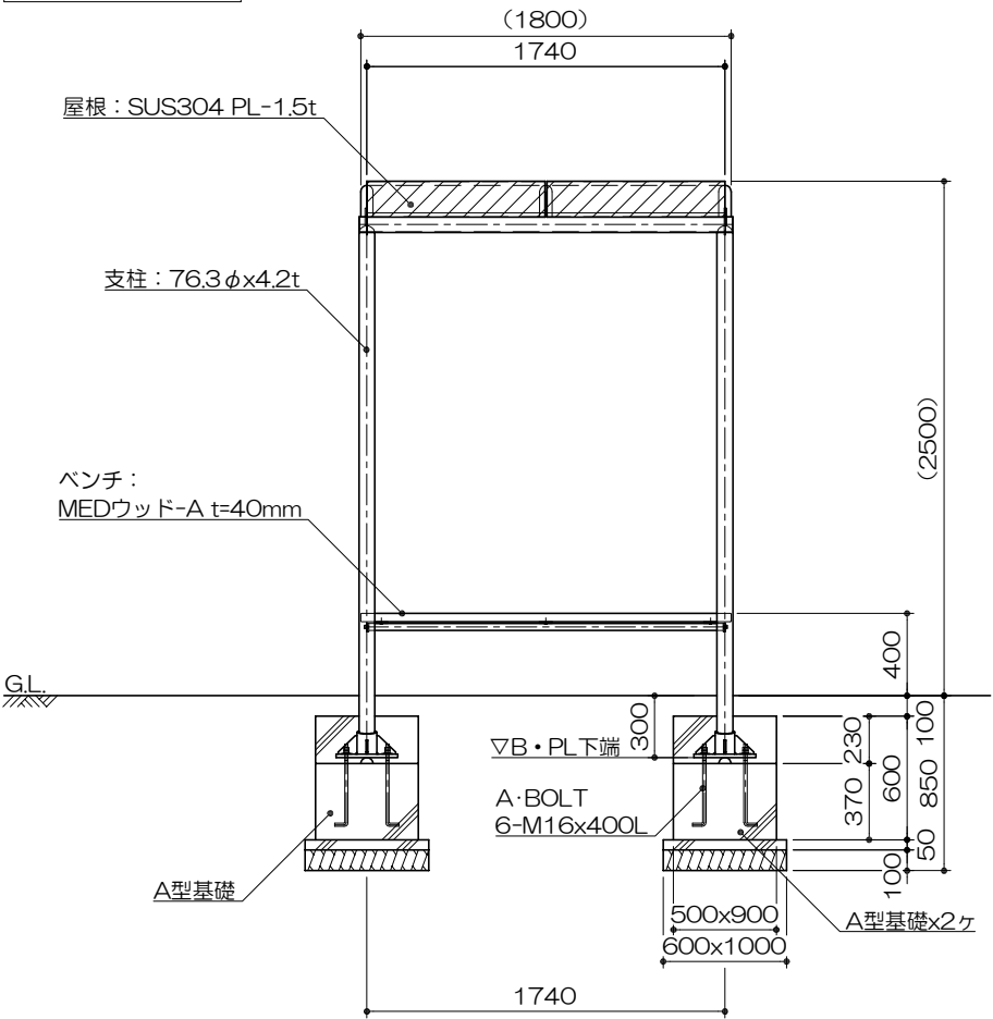
立面図 S= 1 : 40
