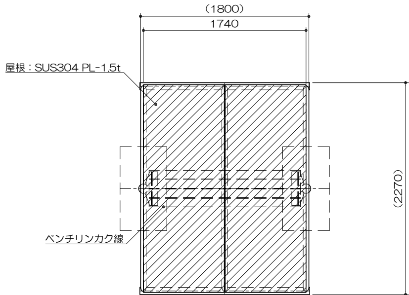
平面図 S= 1 : 40
