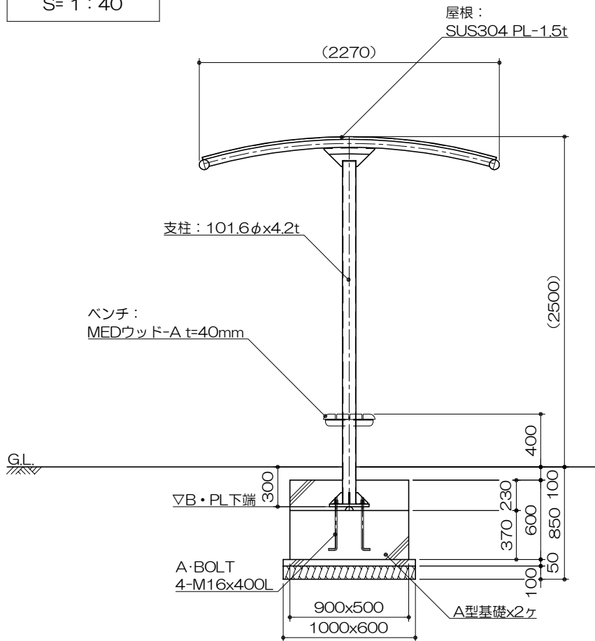
側面図 S= 1 : 40
