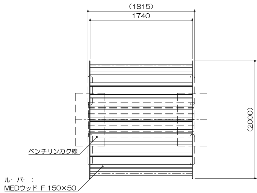
平面図 S= 1 : 40
