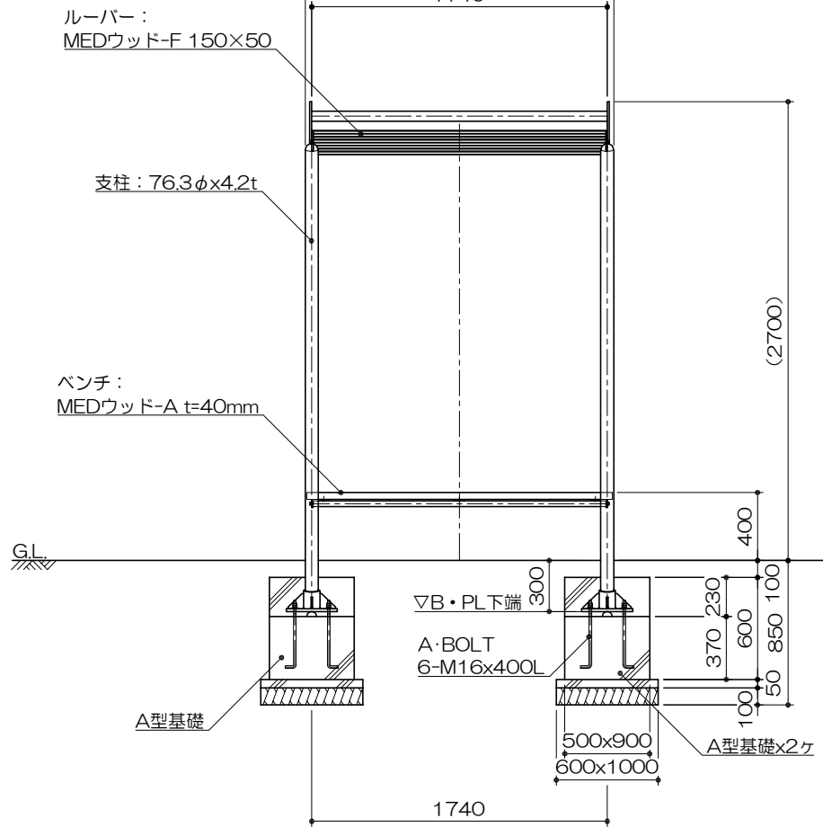
立面図 S= 1 : 40
