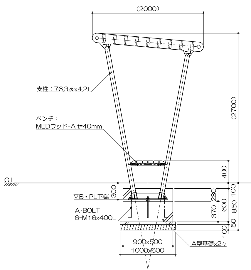
側面図 S= 1 : 40
