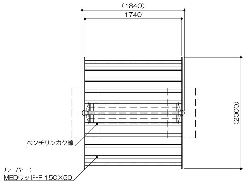
平面図 S= 1 : 40
