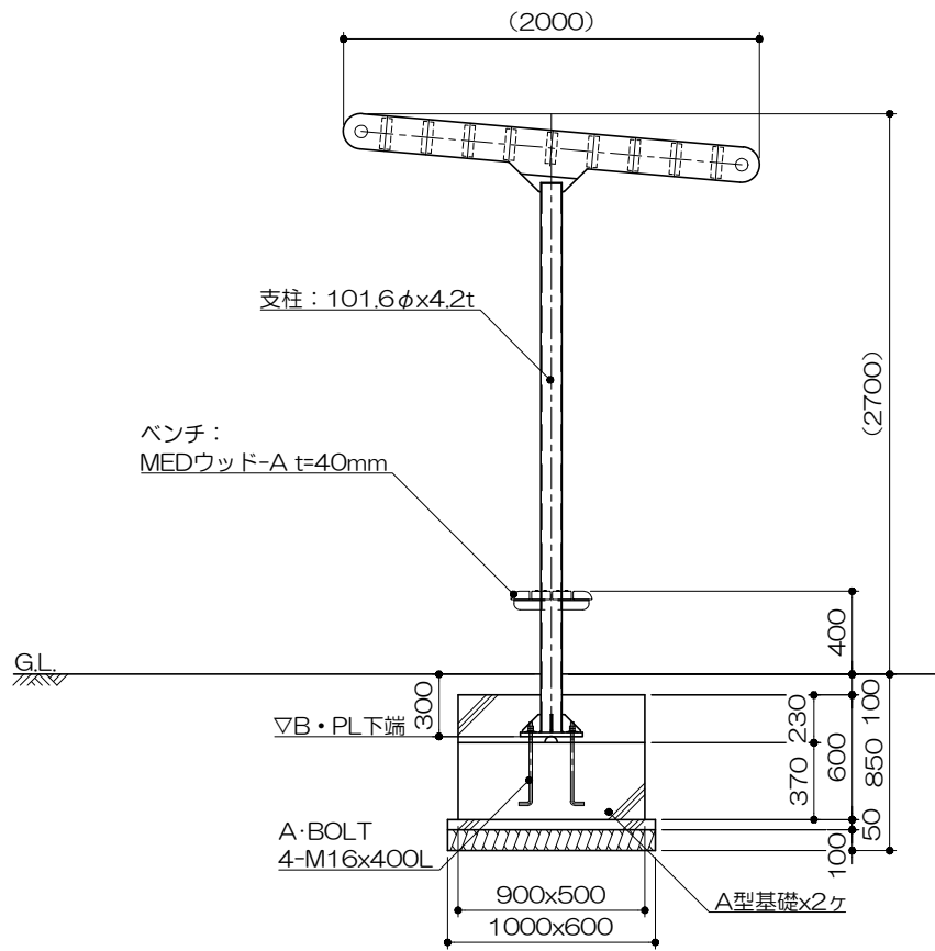
側面図 S= 1 : 40
