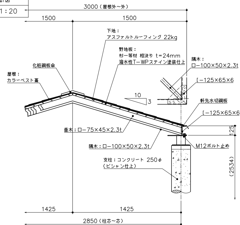
矩計図
