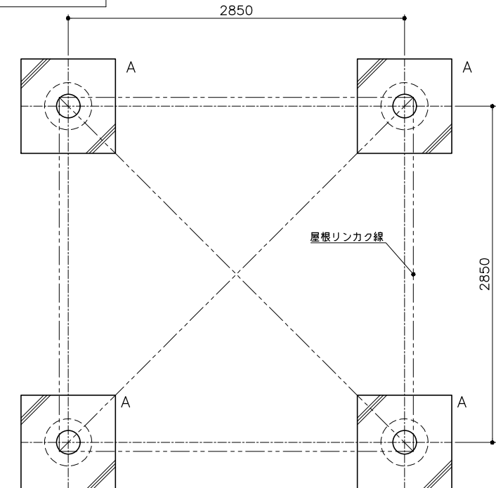
基礎平面図
