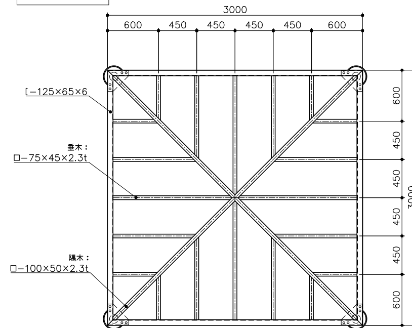
小屋伏図
