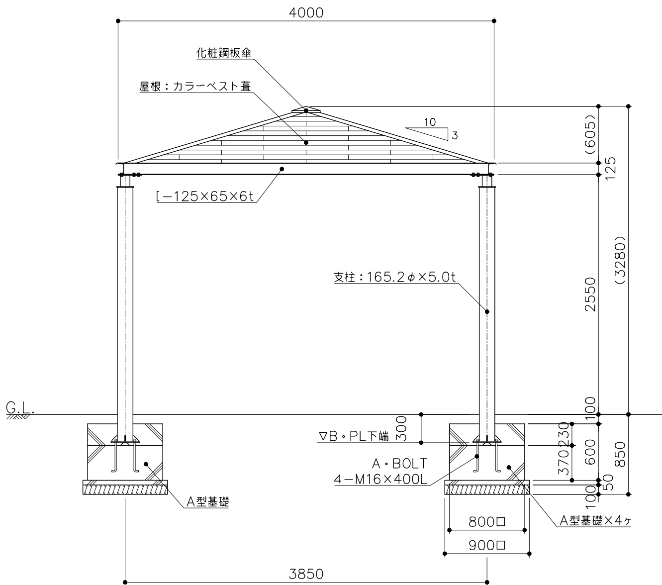
立面図 S= 1:40
