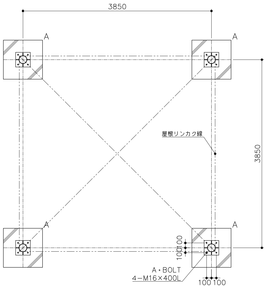
基礎平面図 S= 1:40
