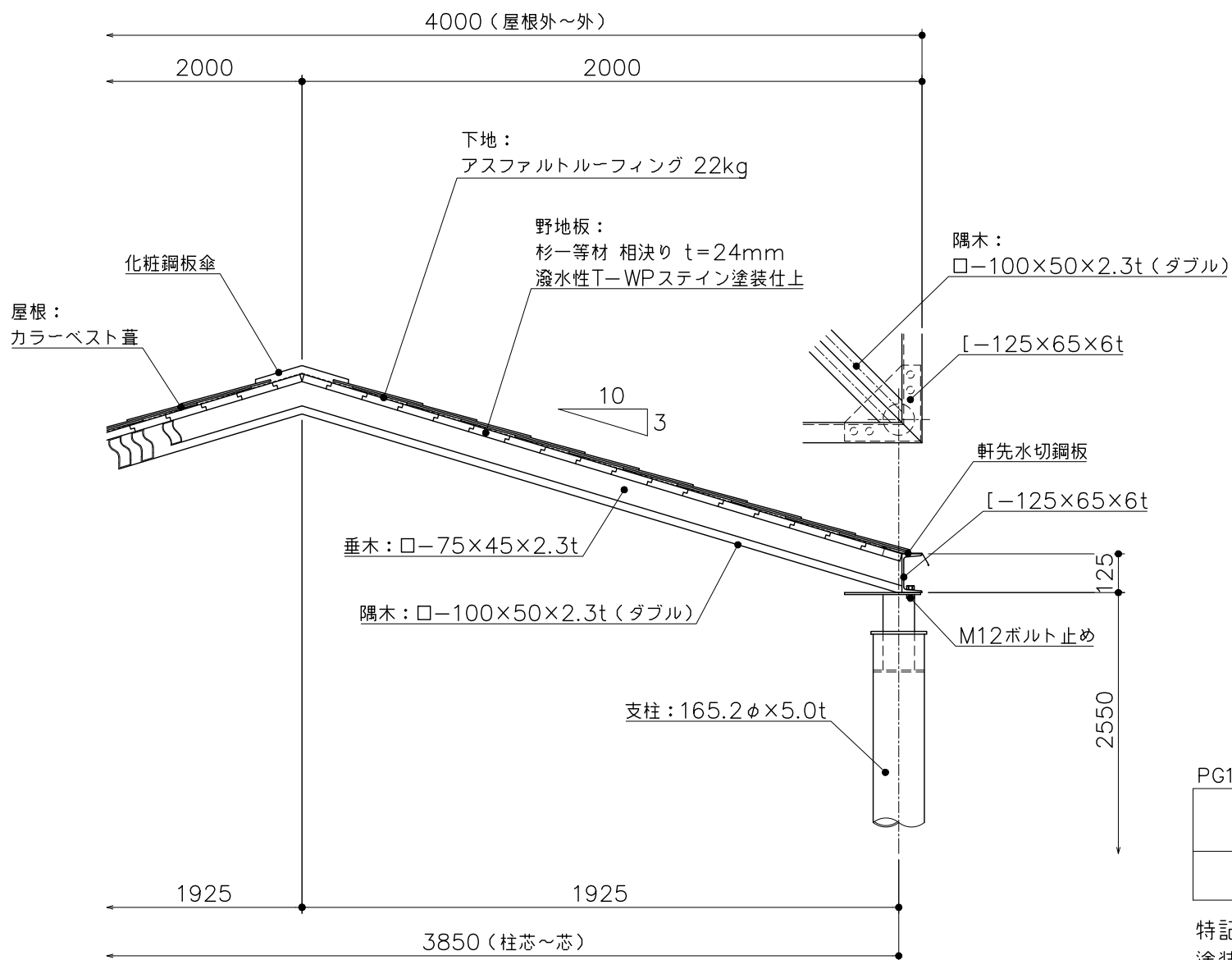
断面図 S= 1:20
