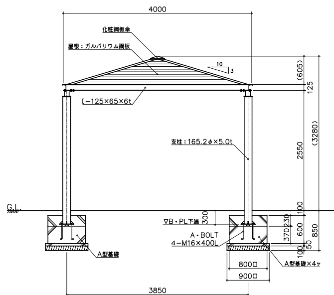
立面図 S= 1: 40
