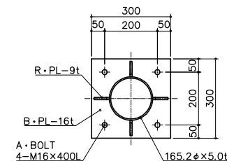
アンカープラン S= 1: 10
