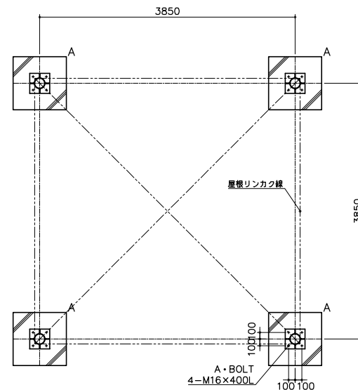
基礎平面図 S= 1: 40
