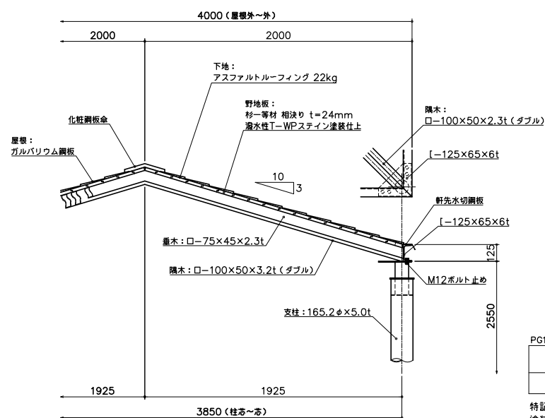
断面図 S= 1: 20
