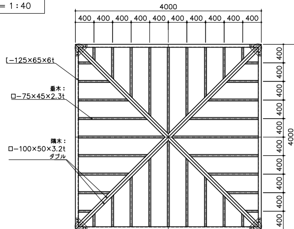
小屋伏図 S= 1: 40
