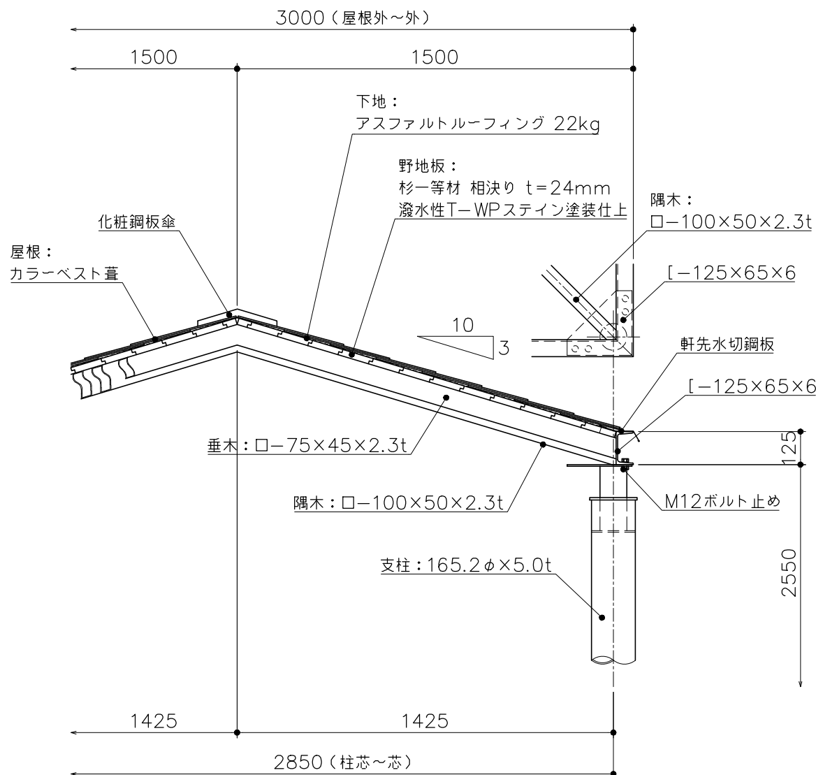
矩計図 S= 1 : 20
