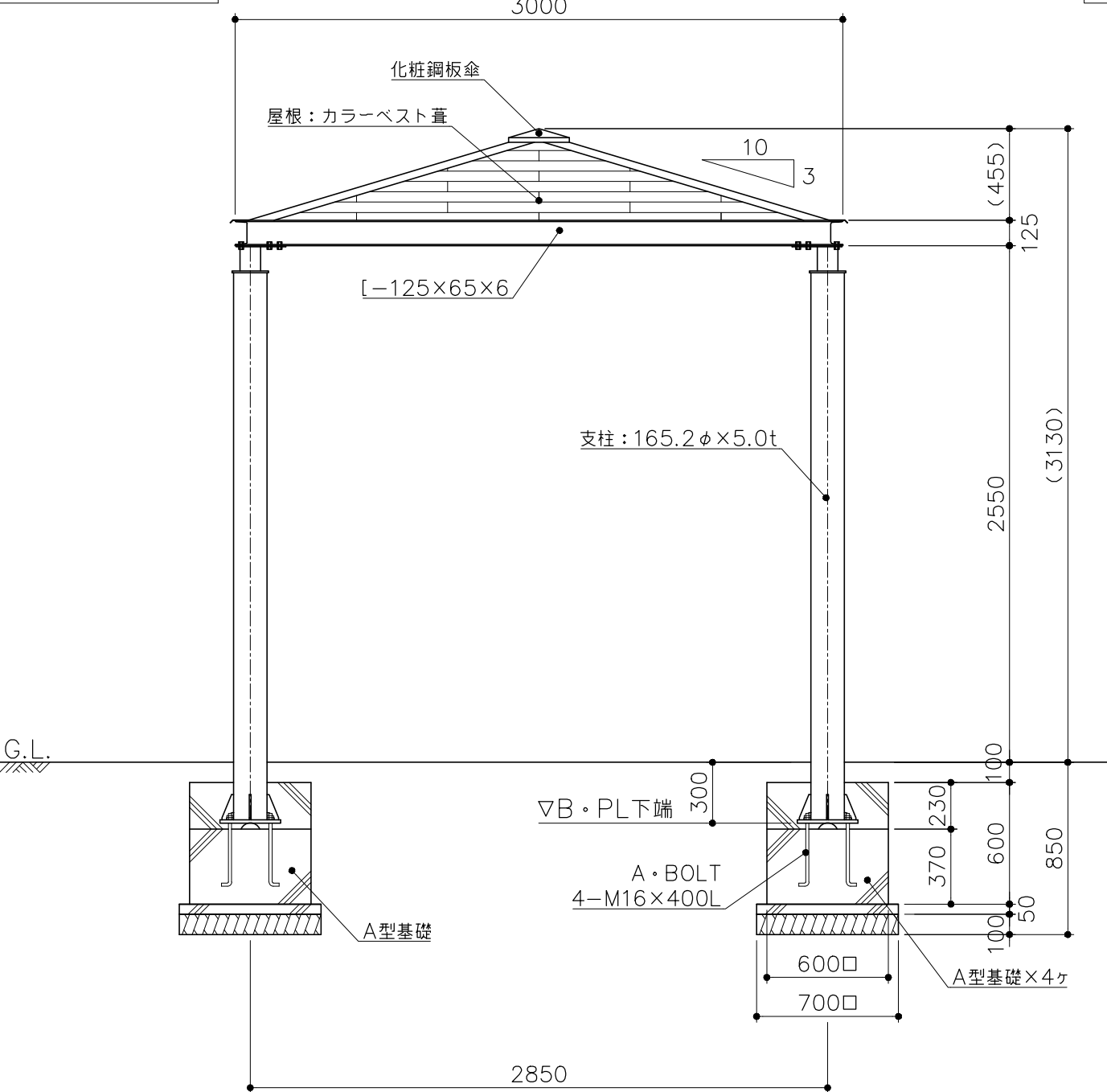
立面図 S= 1 : 30
