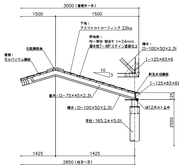
矩計図 S= 1:20
