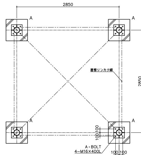
アンカープラン S= 1:10
