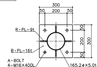
アンカープラン S= 1:10
