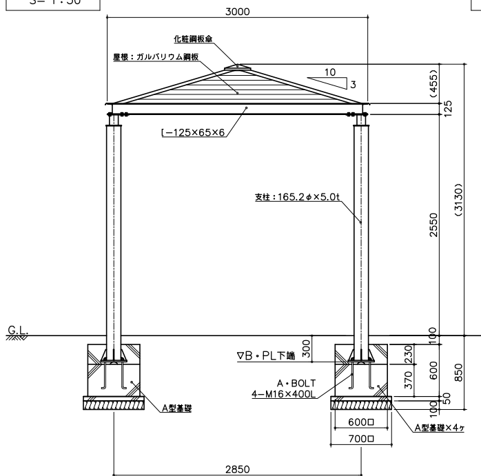
立面図 S= 1:30
