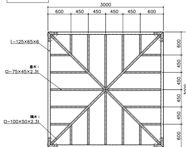
小屋伏図 S= 1:30
