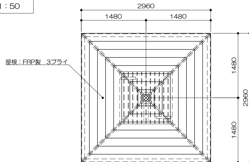
屋根伏図
