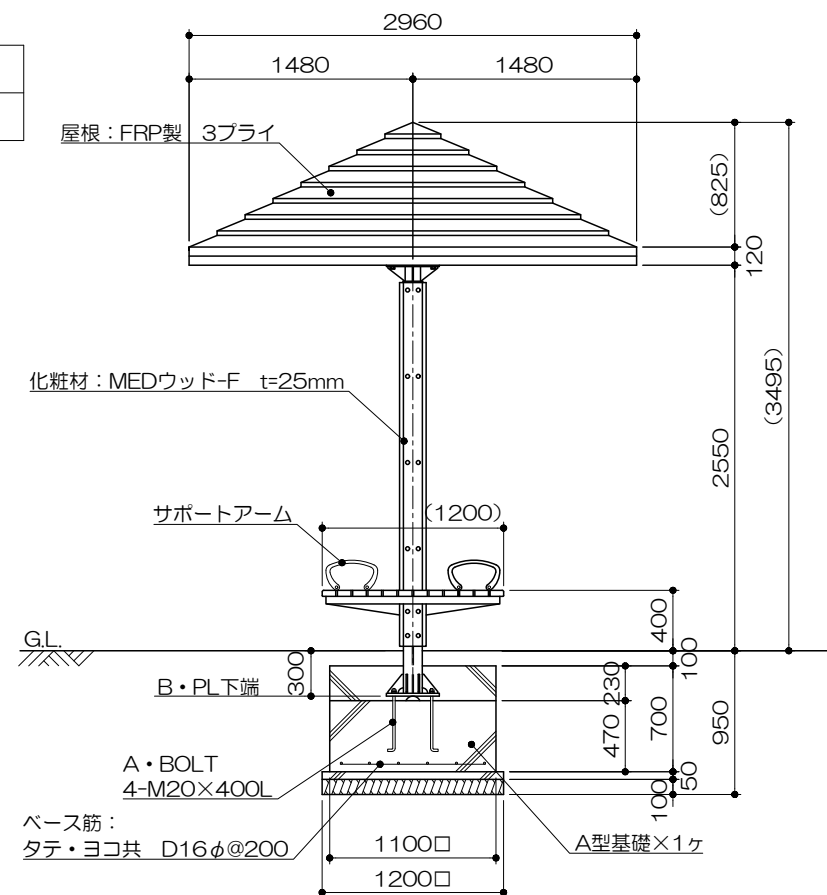
立面图
