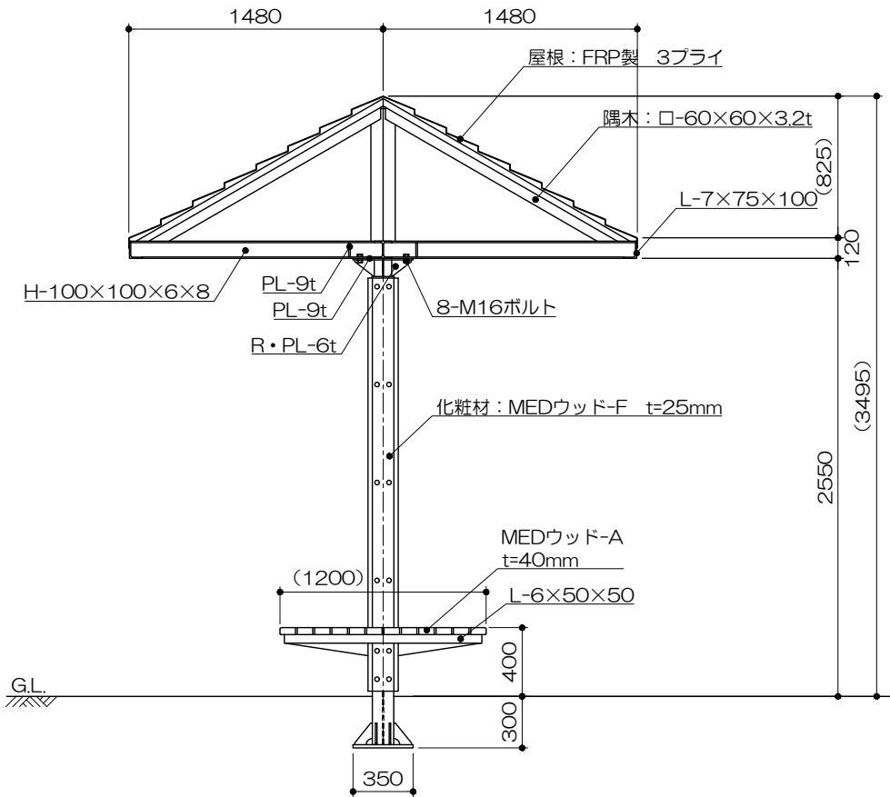
短計図 S= 1 : 40
