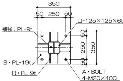
アンカープラン S= 1 : 20
