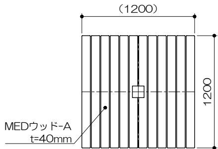
ベンチ平面図 S= 1 : 40
