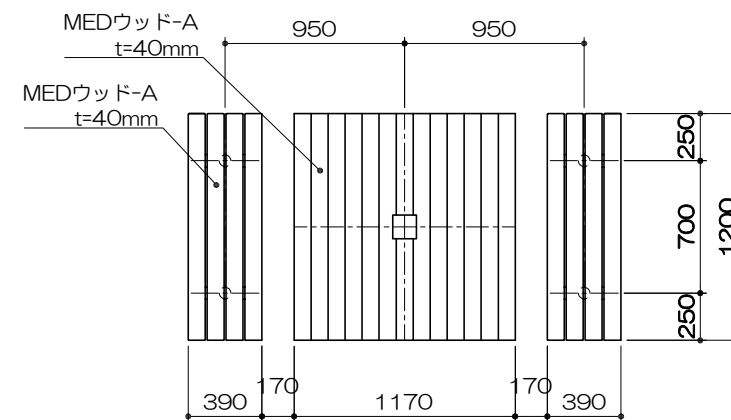
短計図
