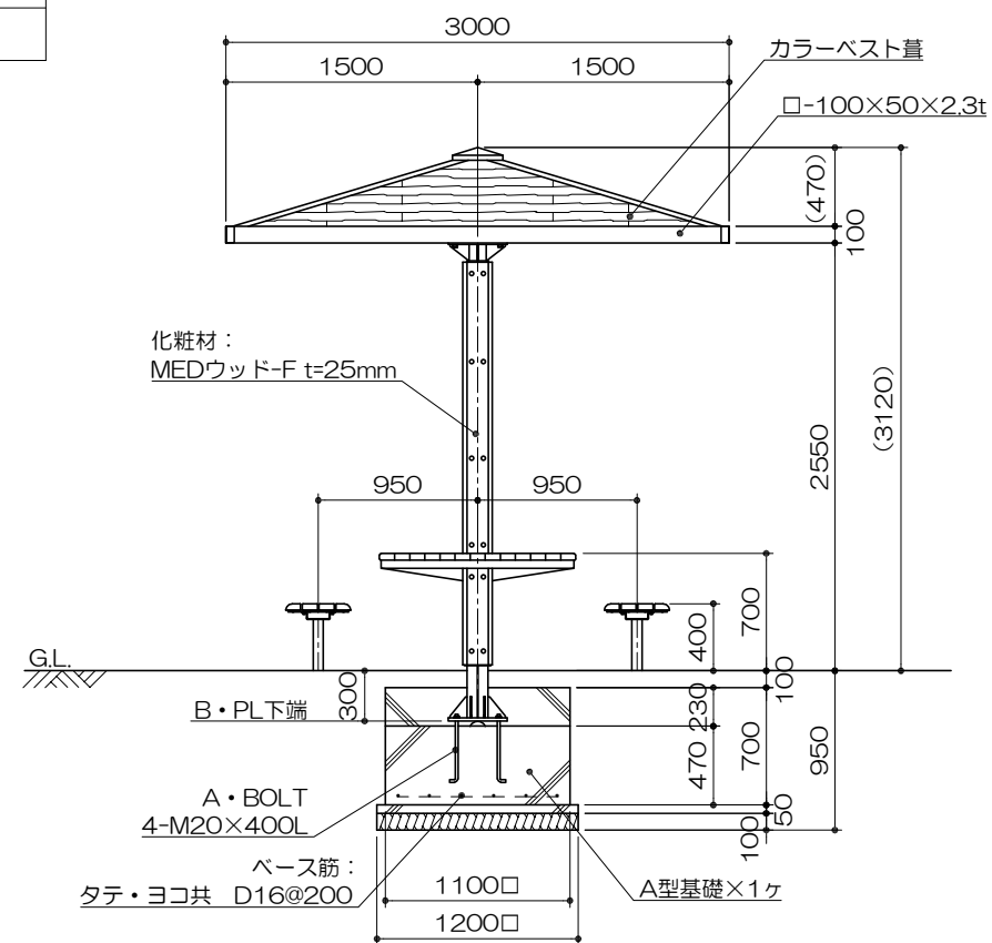
S= 1 : 50
