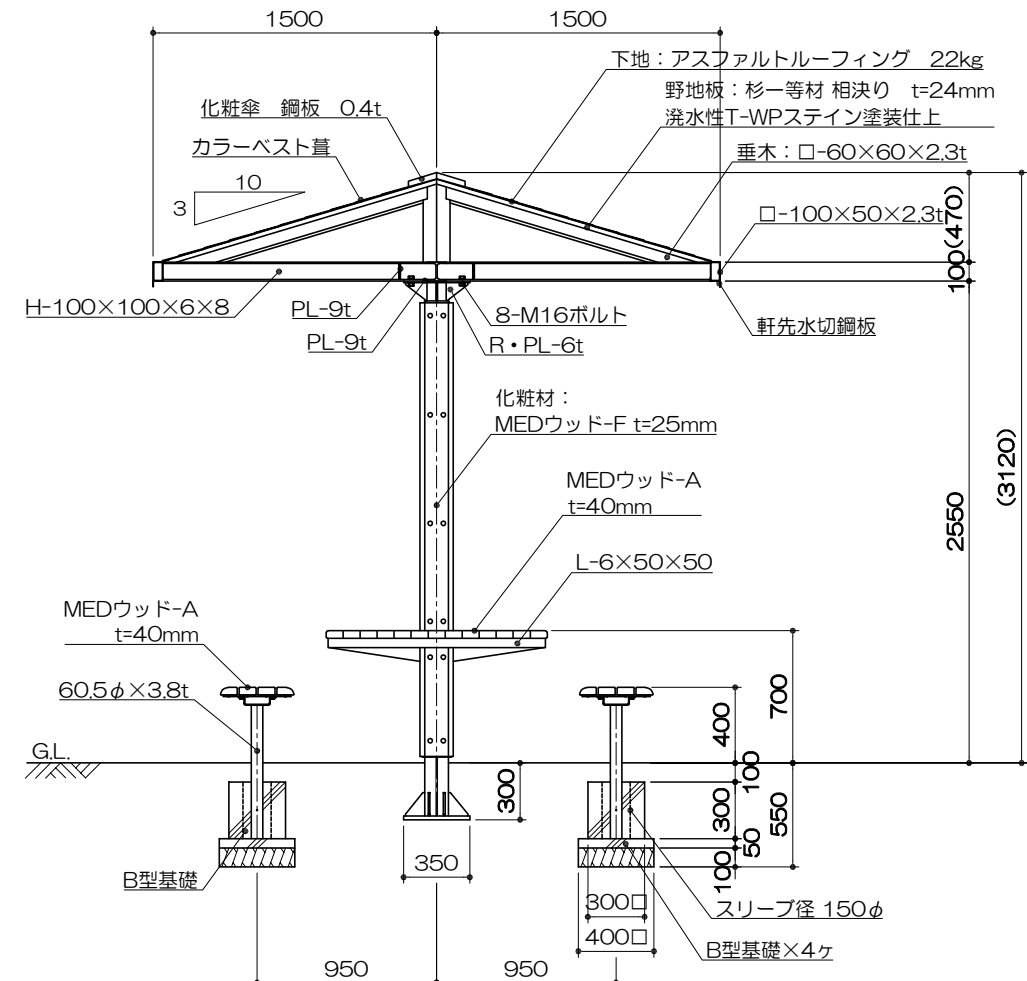
短計図
