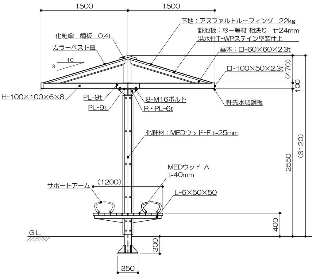
短計図 S= 1 : 40
