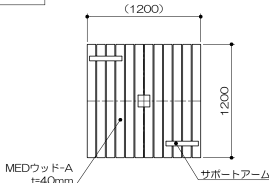
ベンチ平面図 S= 1 : 40
