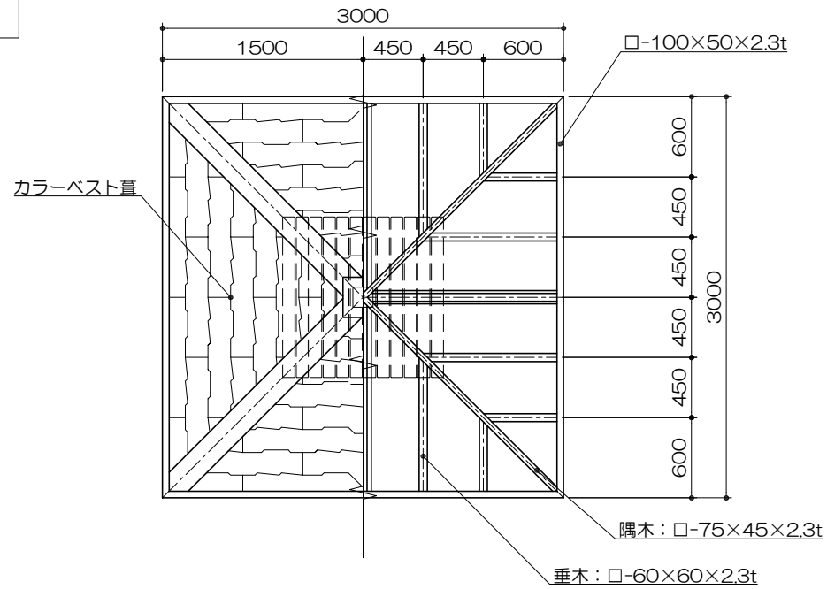
ベンチ平面図 S= 1 : 40
