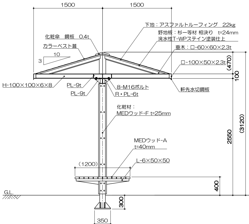
短計図 S= 1 : 40
