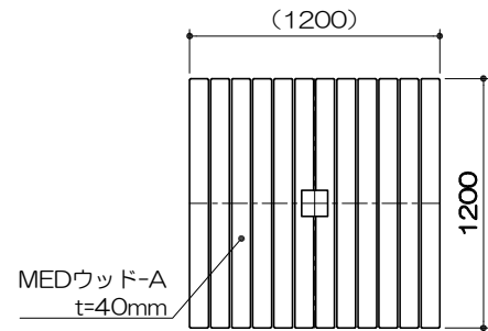
ベンチ平面図 S= 1 : 40
