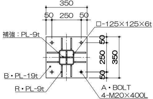
アンカープラン S= 1 : 20
