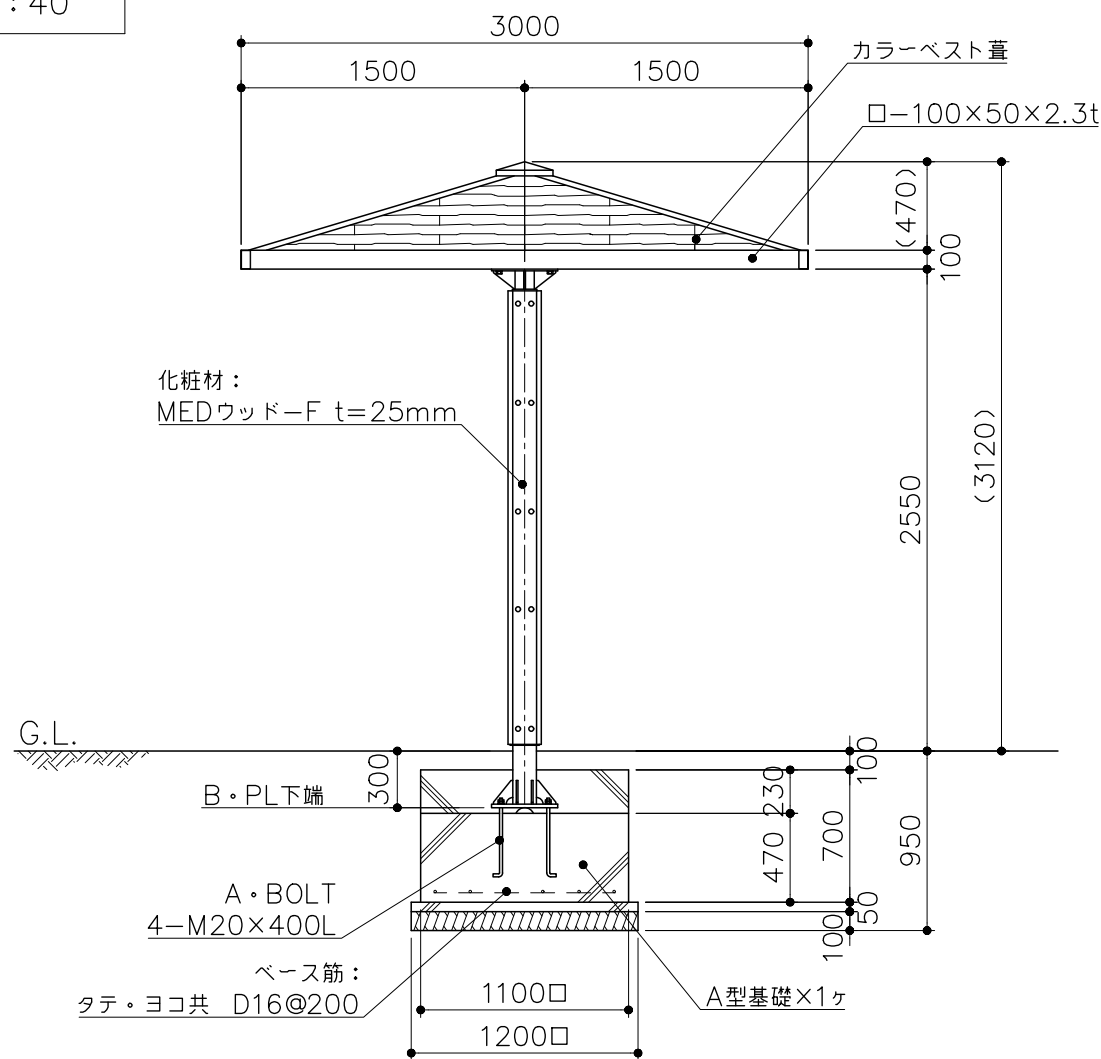
立面図 S= 1 : 40
