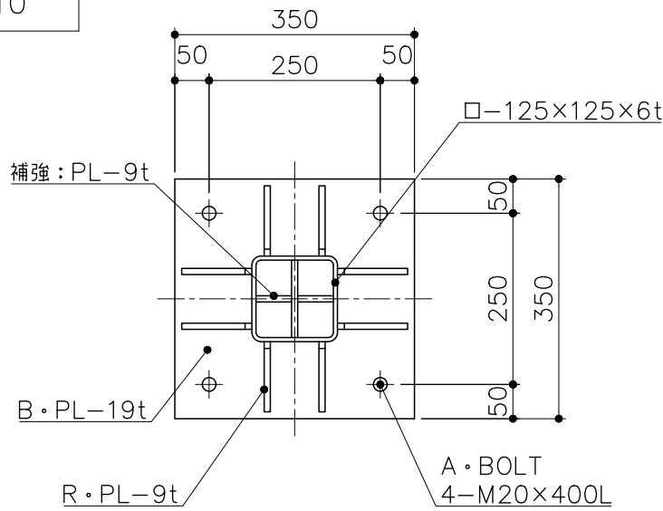
アンカープラン S= 1 : 10
