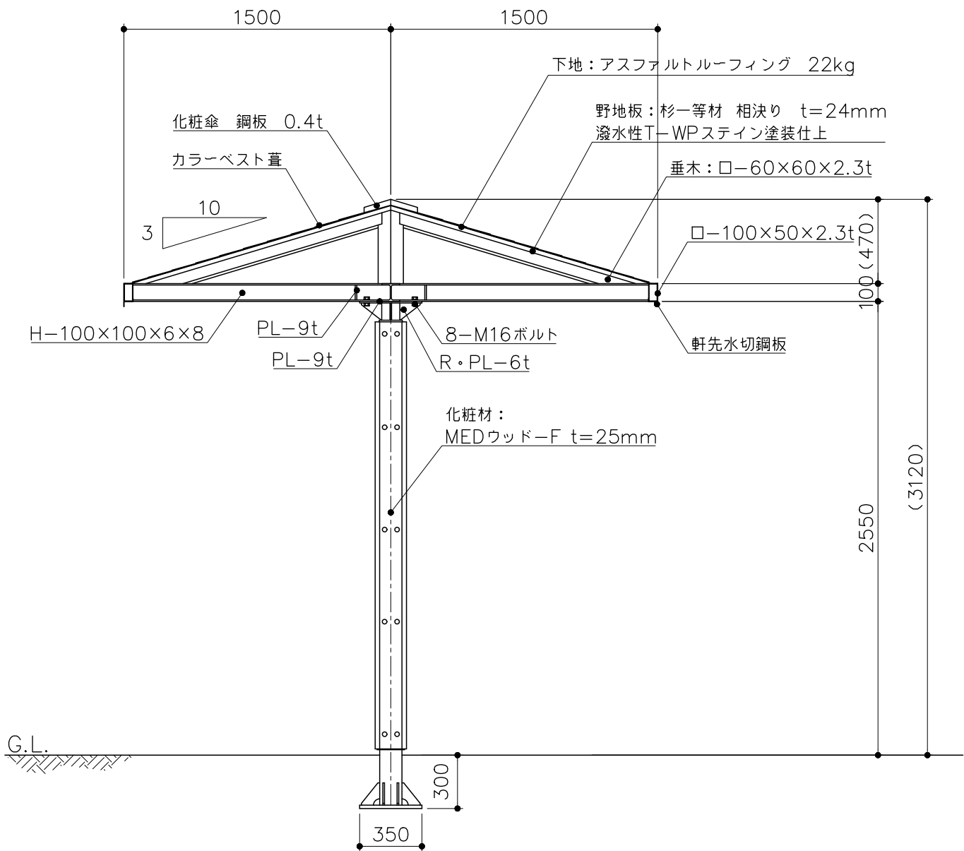
矩計図 S= 1 : 30
