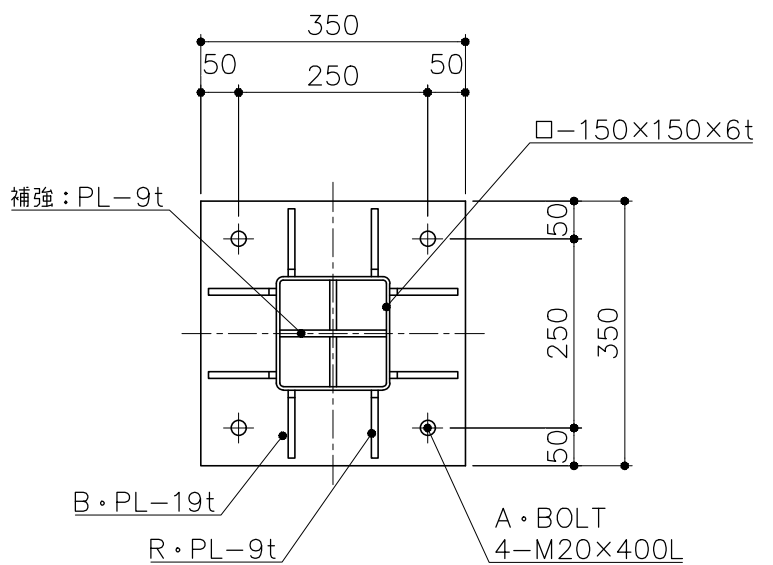
アンカープラン S= 1 : 10
