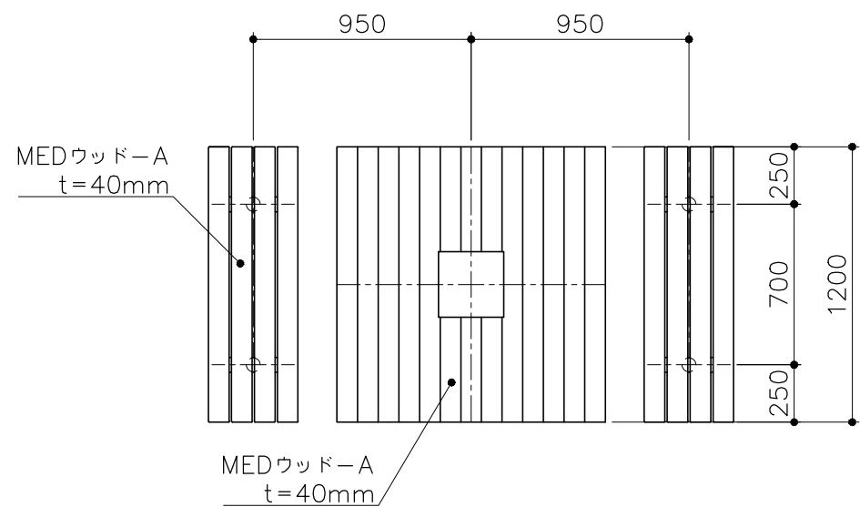
テーブル・ベンチ平面図 S= 1 : 30
