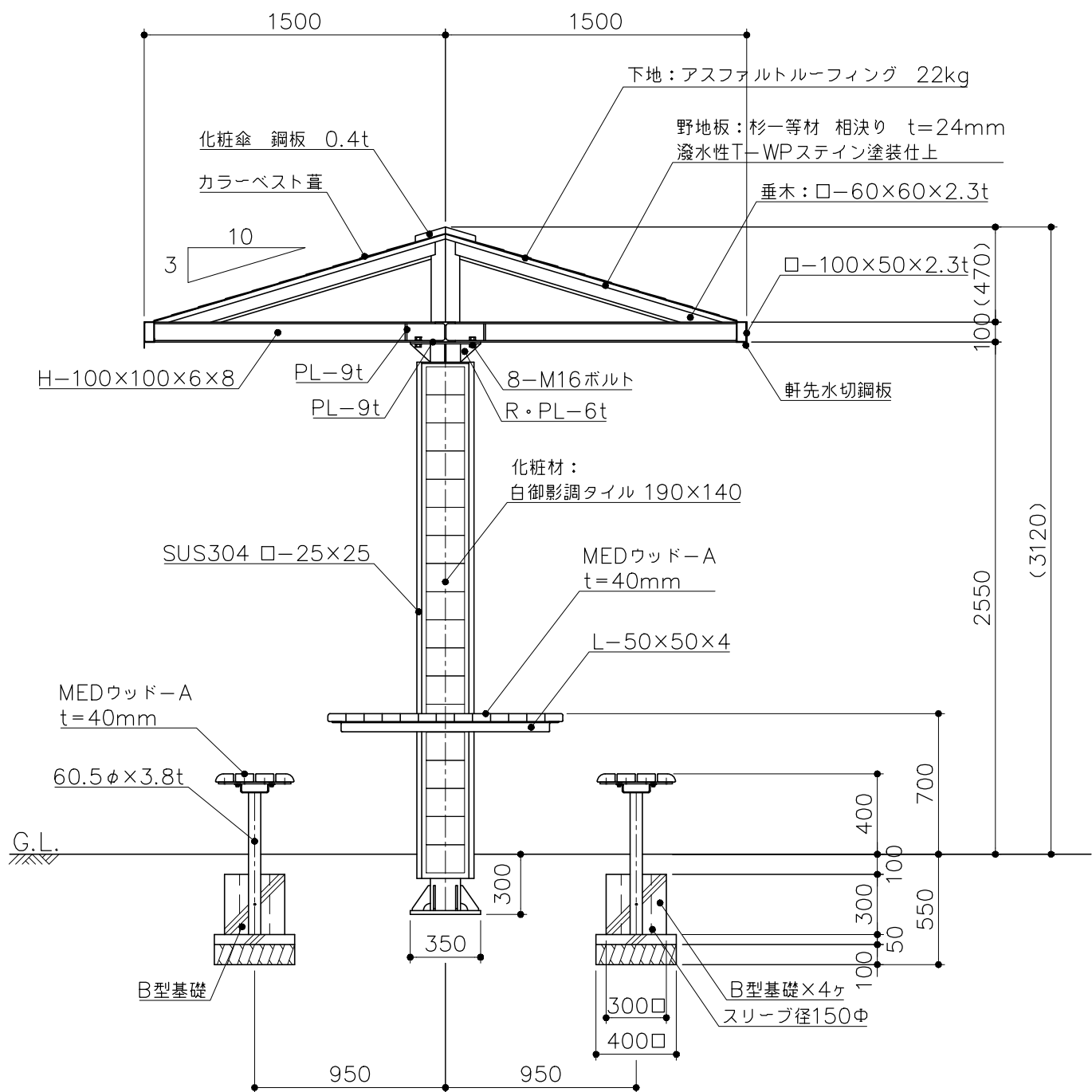
矩計図 S= 1 : 30
