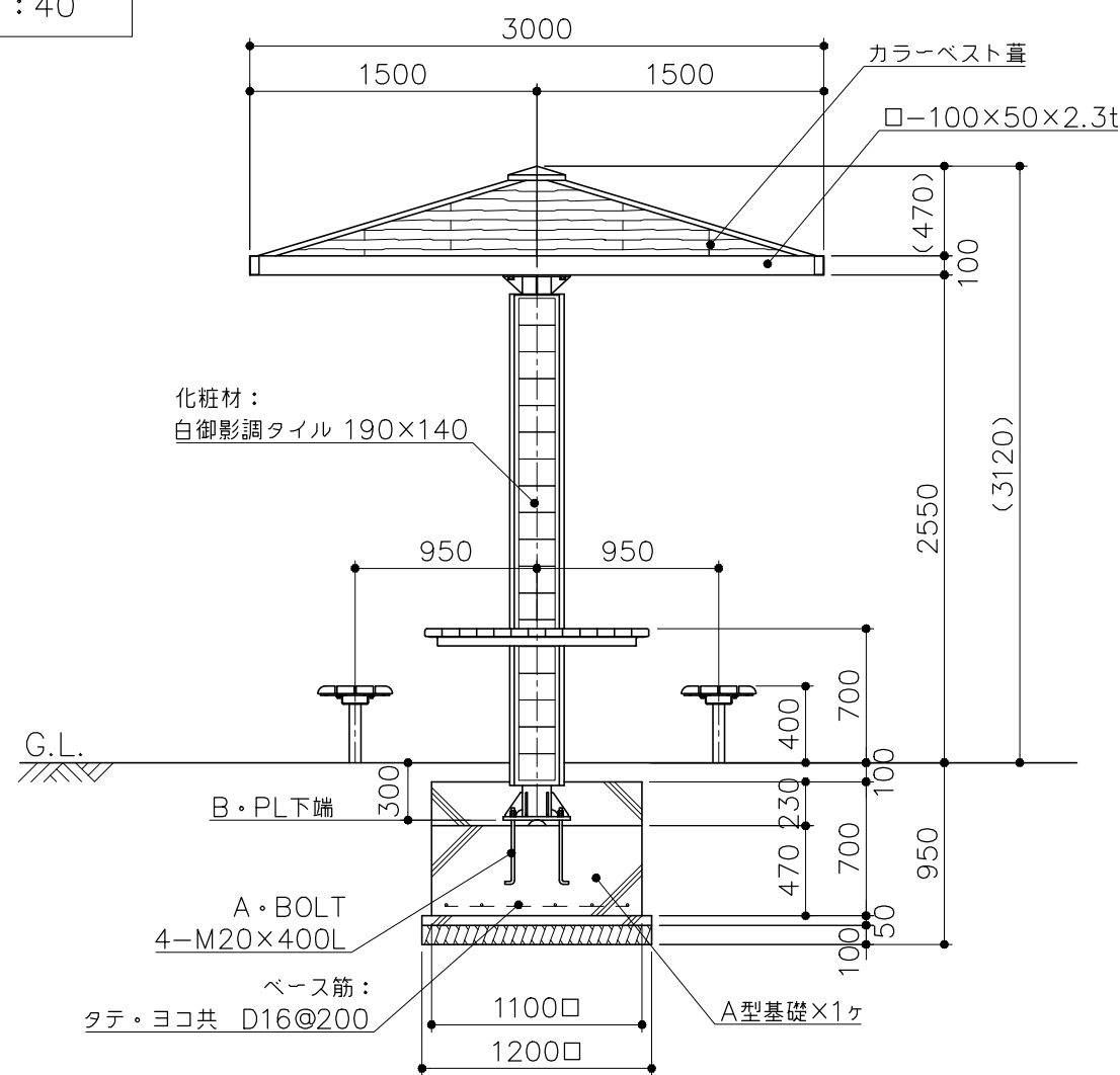
立面図 S= 1 : 40
