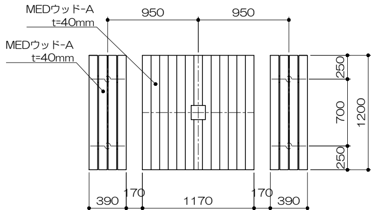
短計図 S= 1 : 40
