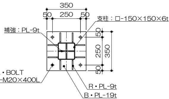
アンカープラン S= 1 : 20
