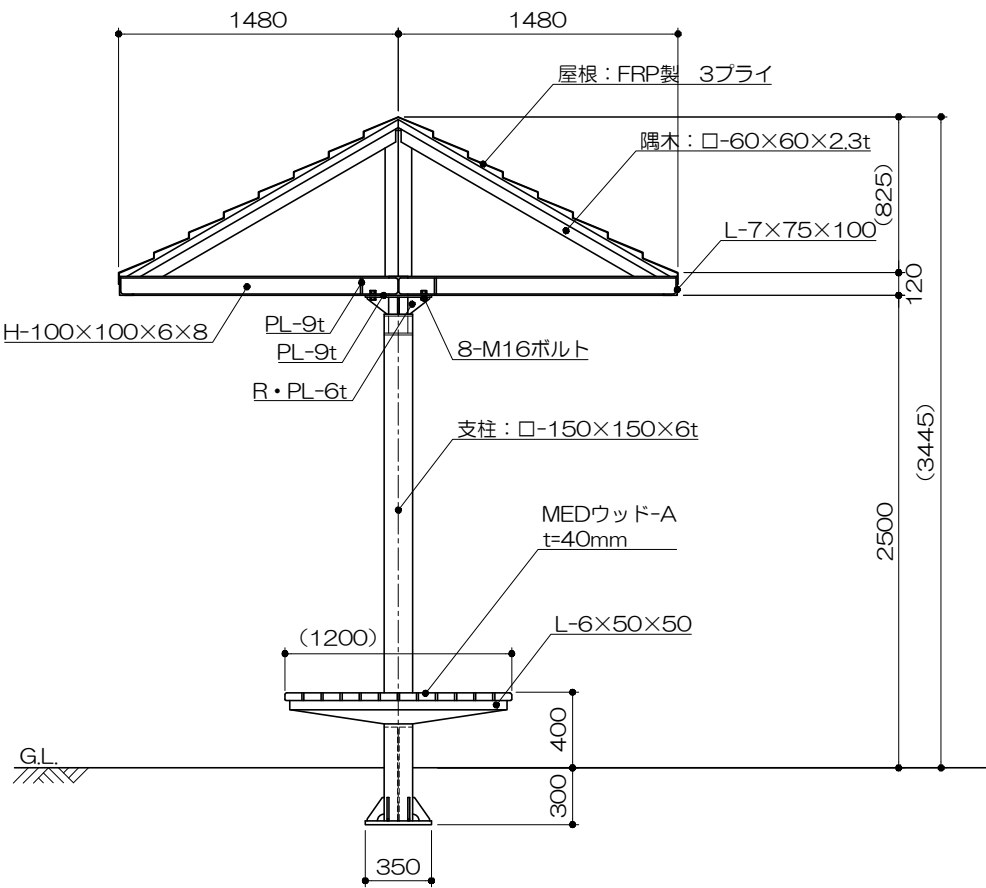
短計図 S= 1 : 40
