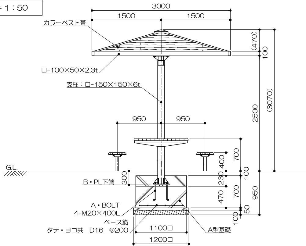
基礎平面図 S= 1 : 50
