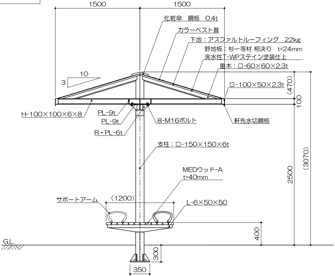
短計図 S= 1 : 40
