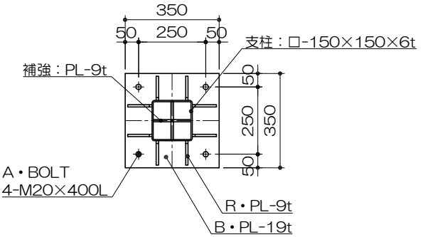
アンカープラン S= 1 : 20
