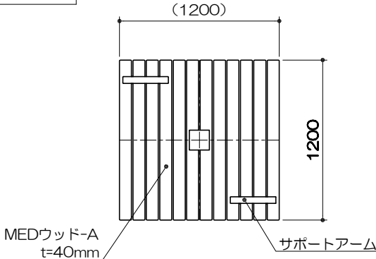
ベンチ平面図 S= 1 : 40
