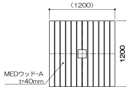
ベンチ平面図
