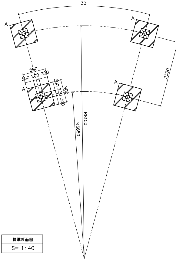
基礎平面図 S= 1:40
