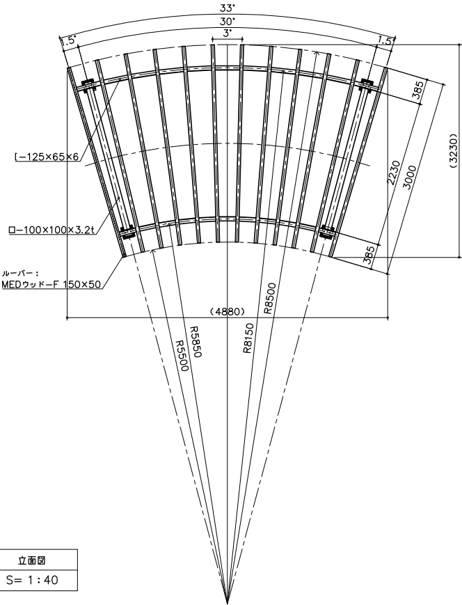
平面図 S= 1:40
