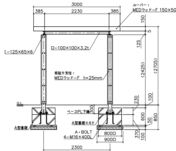
標準断面図 S= 1:40
