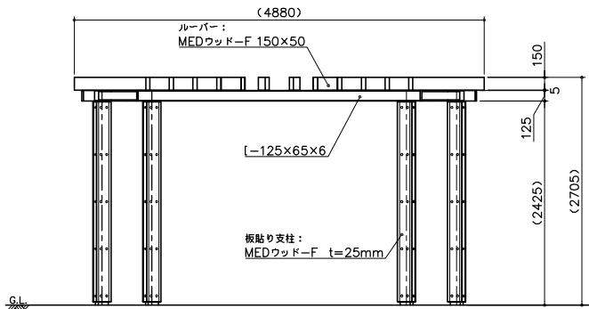
立面図 S= 1:40
