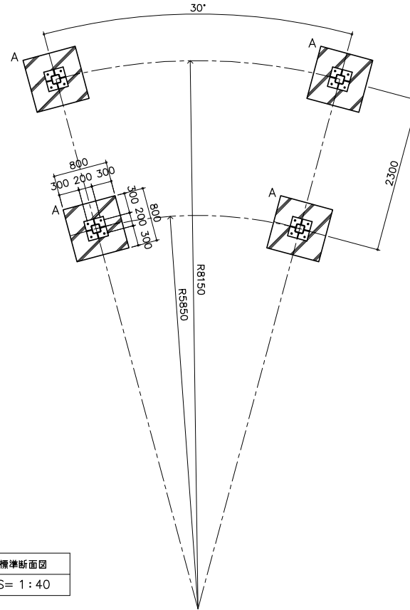
基礎平面図 S= 1:40
