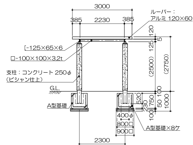
立面图 S= 1 : 100
