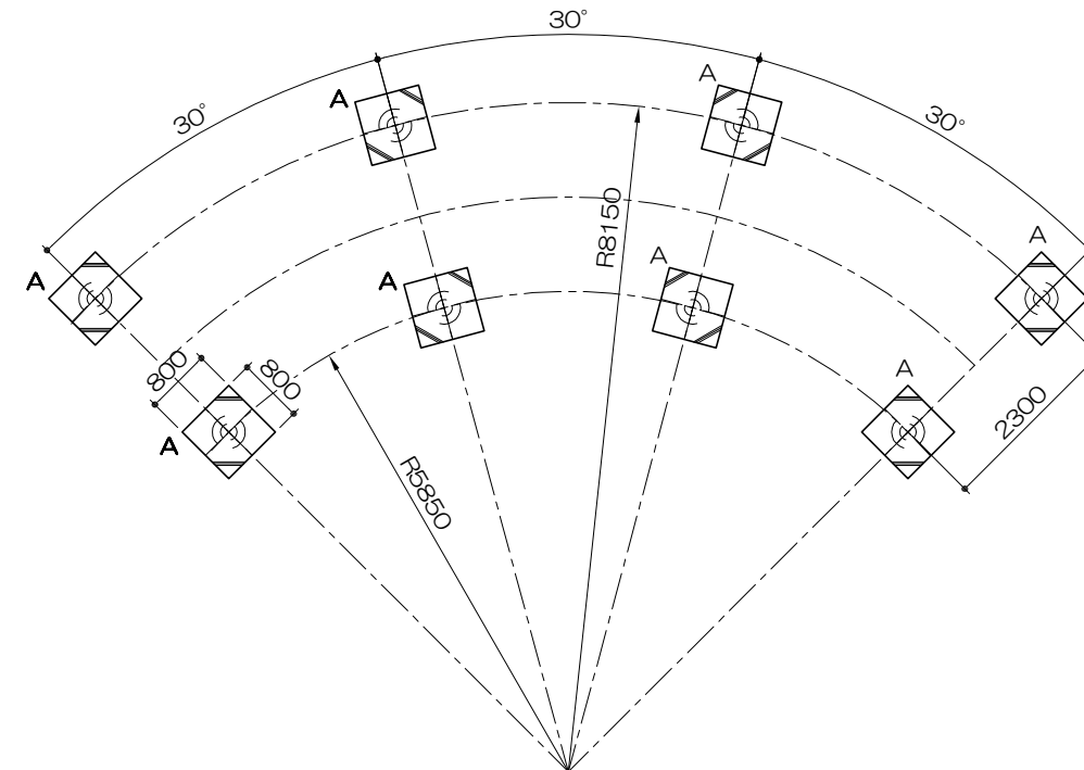
基礎平面図 S= 1 : 100
