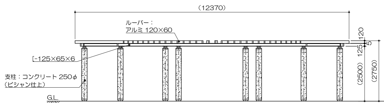
立面图 S= 1 : 100
