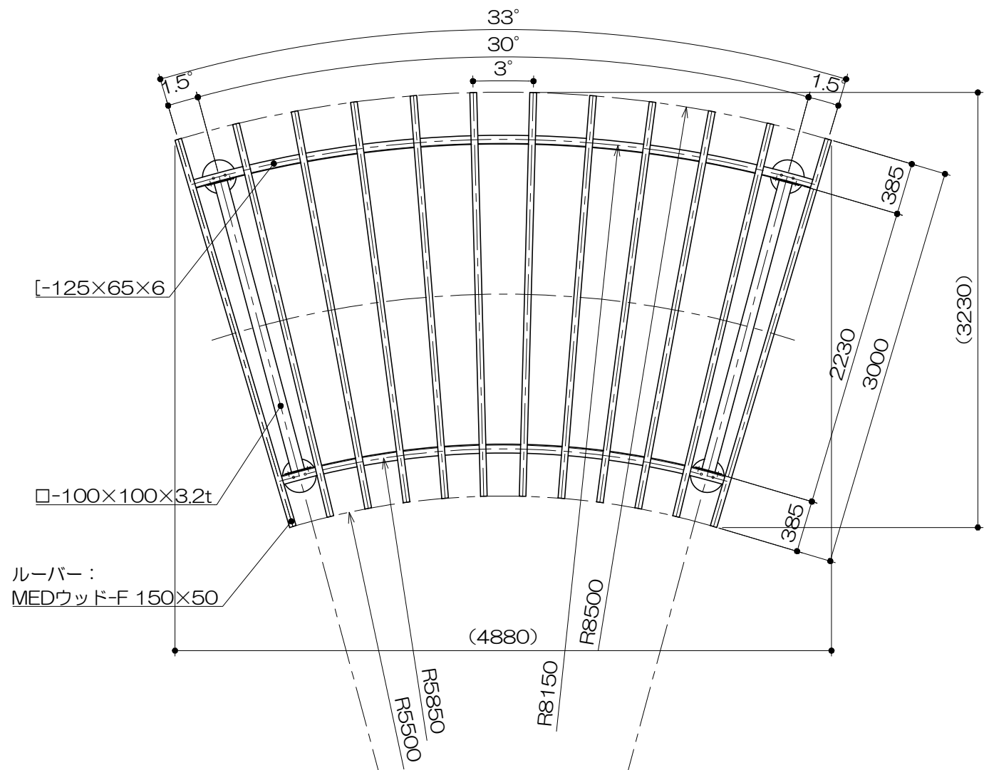
平面図 S= 1 : 40
