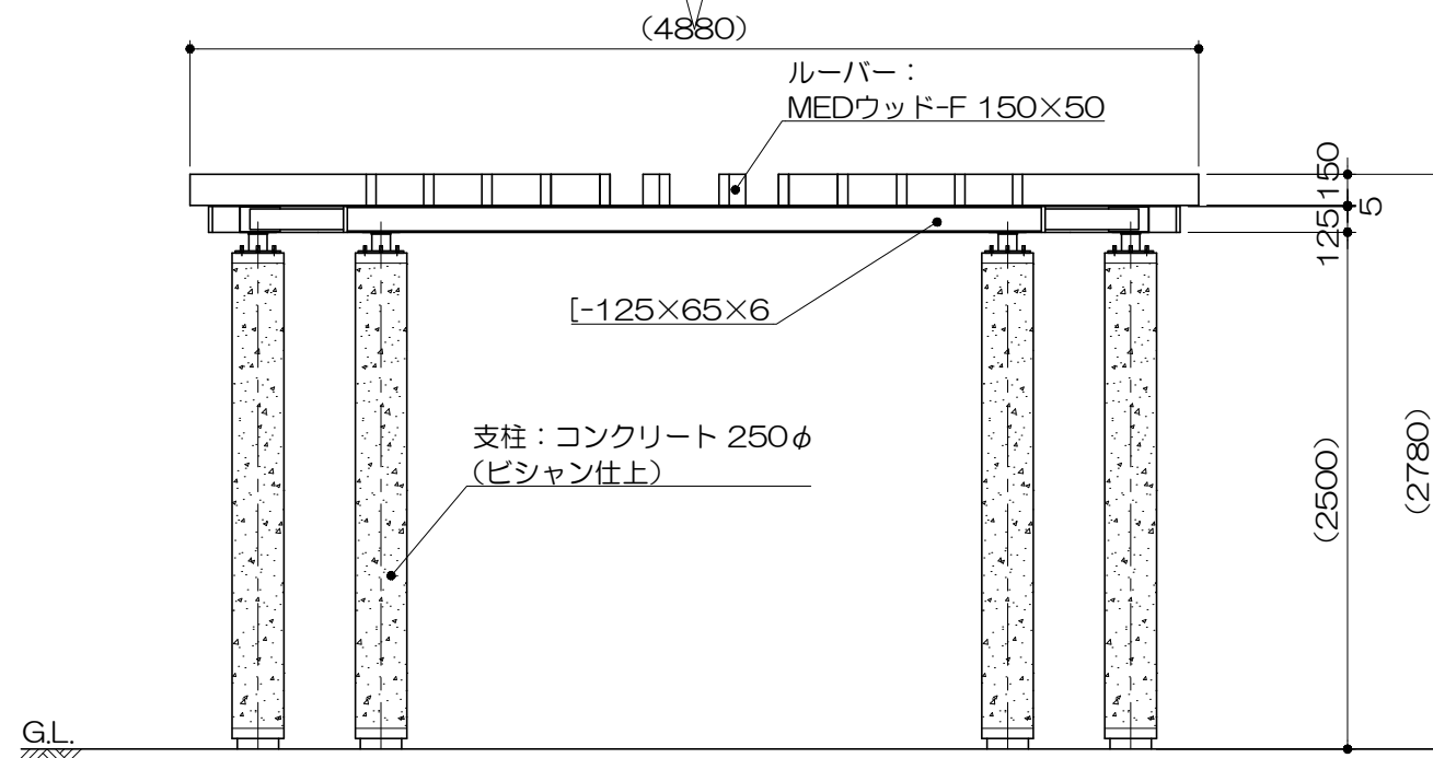
立面図 S= 1 : 40
