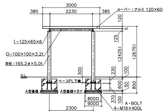
(12370) ルーバー: アルミ 120×60 〔-125×65×6〕 支柱: 165.2φ×5.0t 120 5 125 (2425) (2675)
