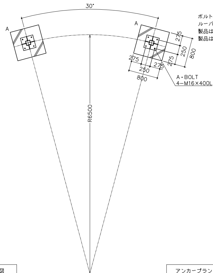
アンカープラン
