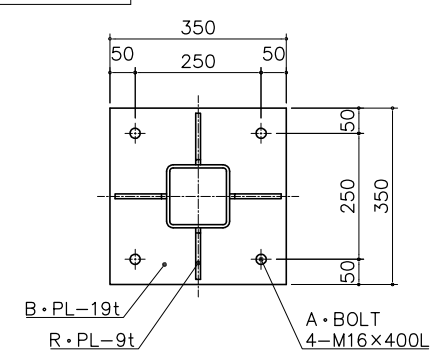
アンカープラン
