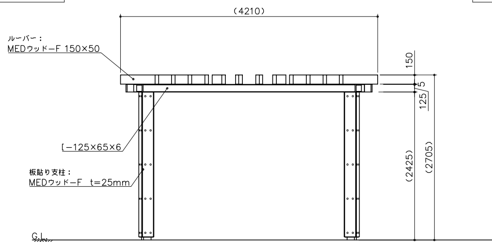
立面图
