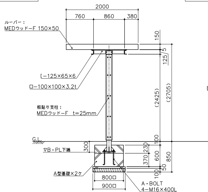
標準断面図
