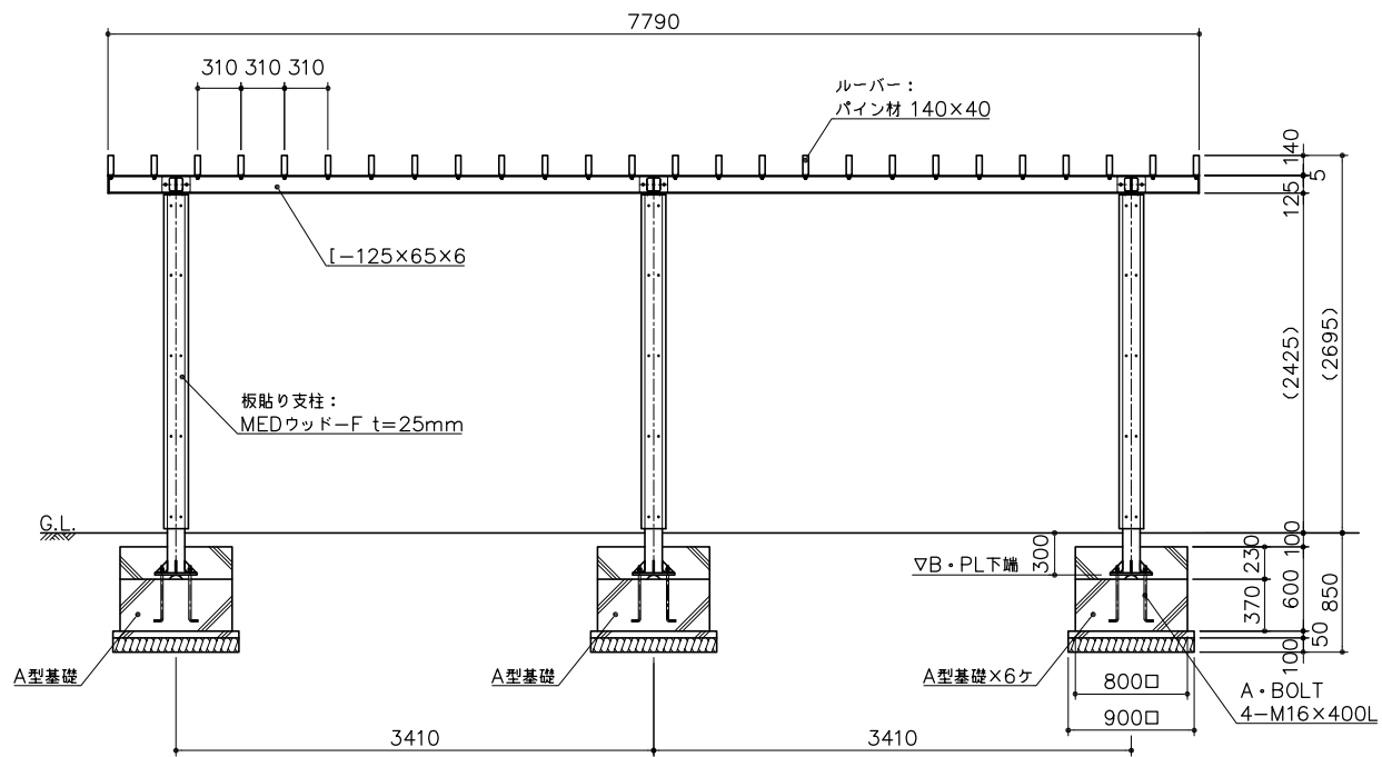
立面図 S= 1 : 40
