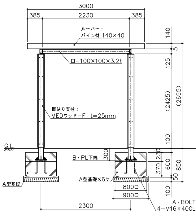
側面図 S= 1 : 40
