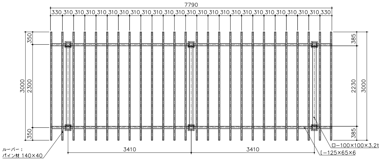
平面図 S= 1 : 40
