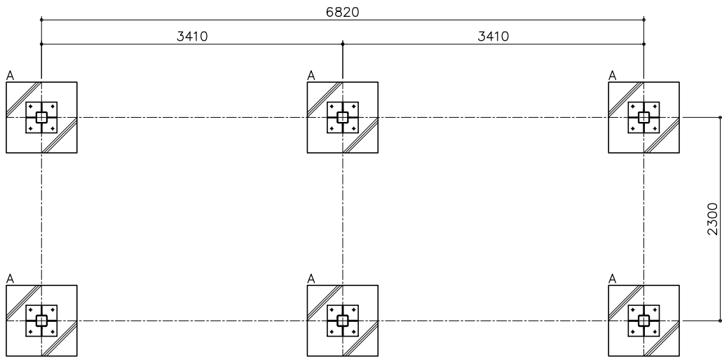
基礎平面図 S= 1 : 40
