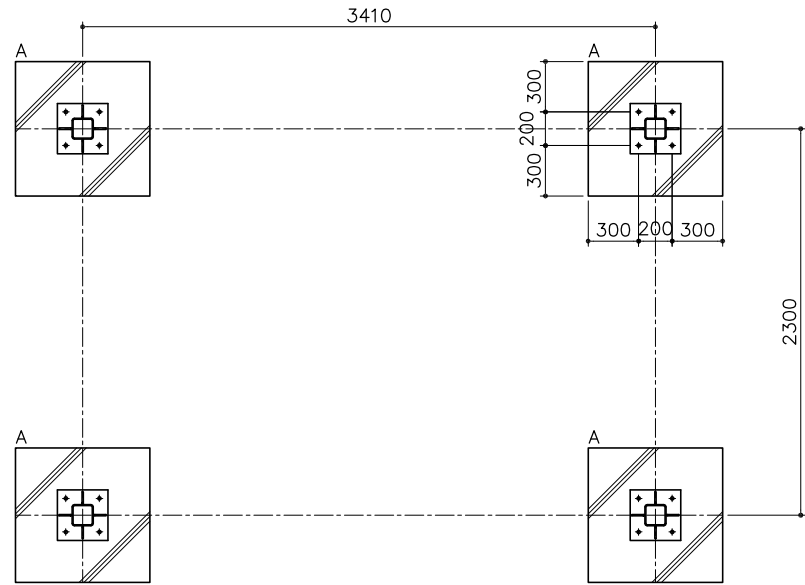
基礎平面図 S= 1 : 30
