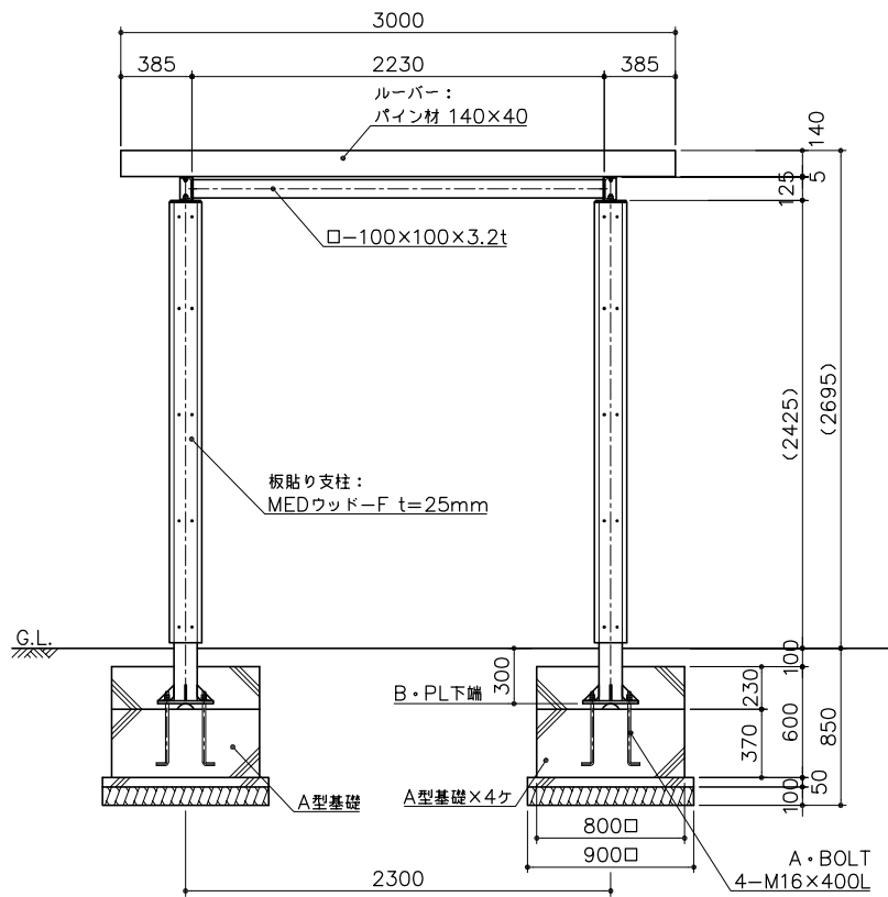
側面図 S= 1 : 30
