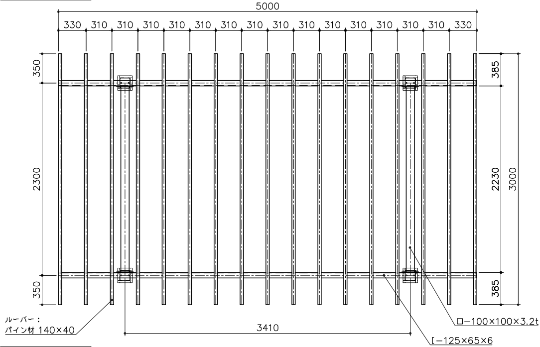
立面図 S= 1 : 30
