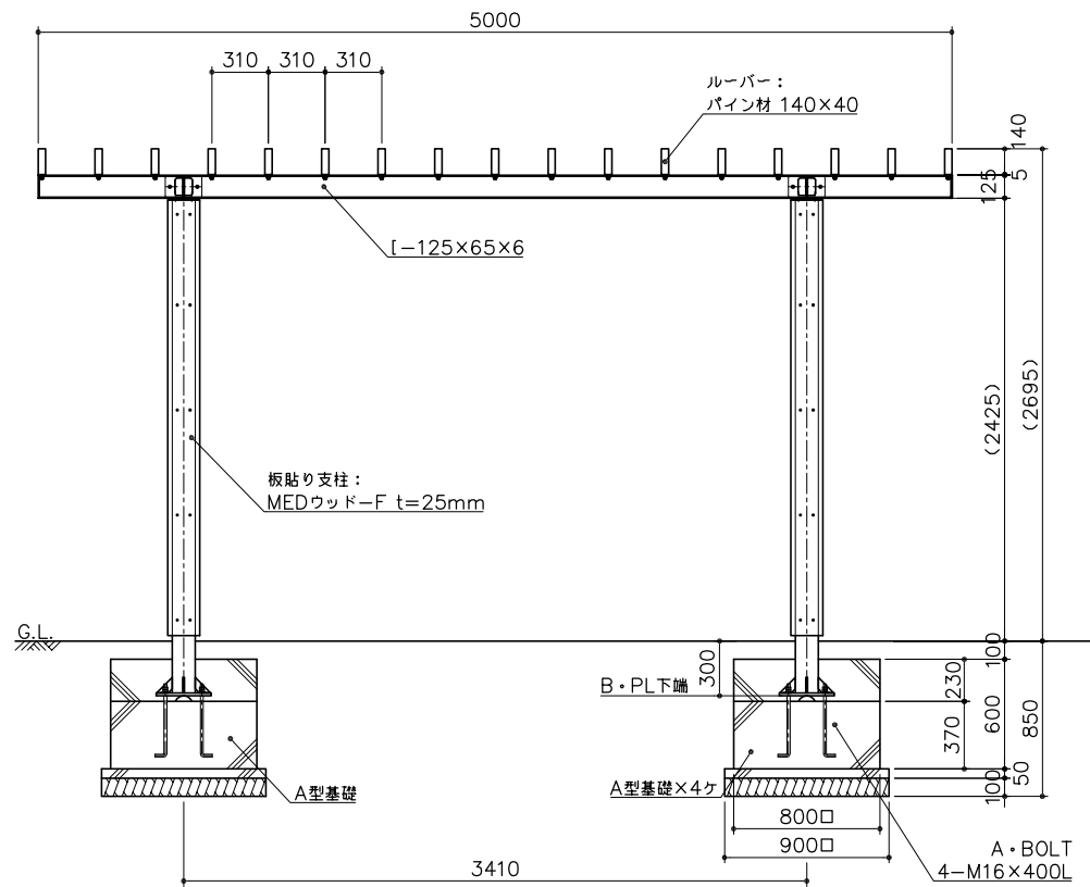
立面図 S= 1 : 30
