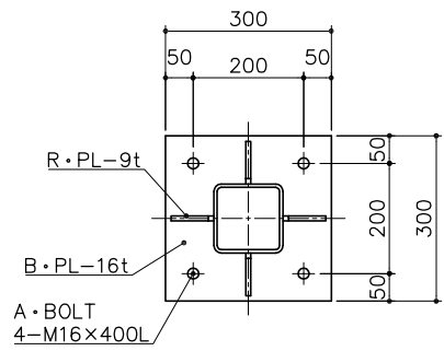
アンカープラン S= 1 : 10
