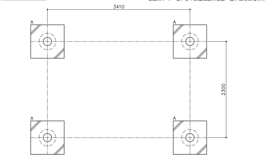
基礎平面図 S= 1:30
