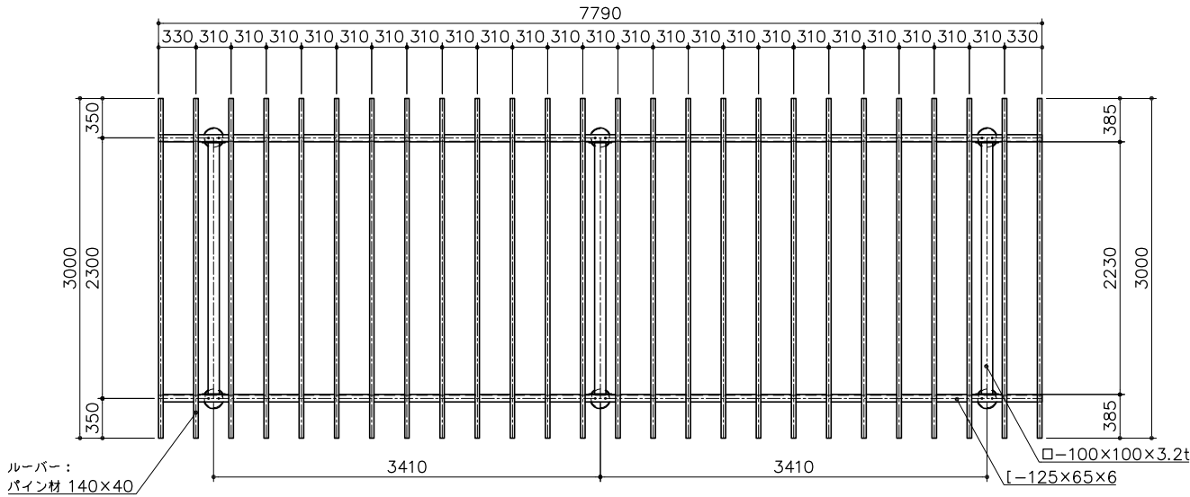
平面図 S＝ 1：40
