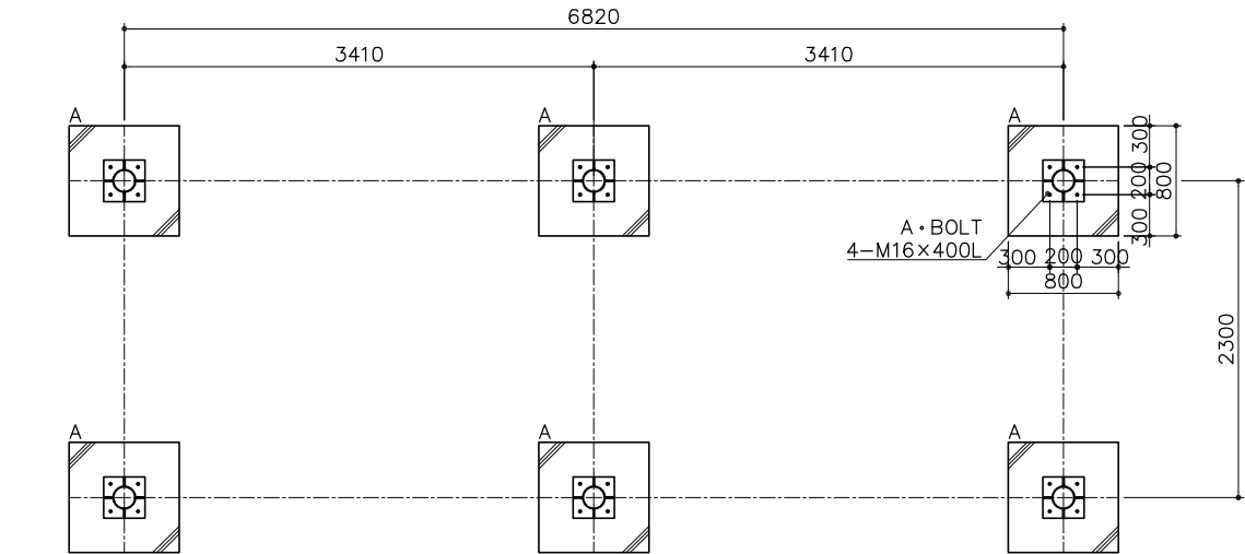
基礎平面図 S＝ 1：40
