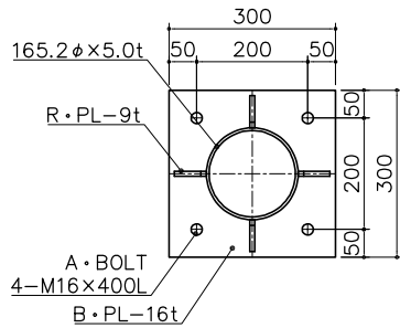
アンカープラン S＝ 1：10
