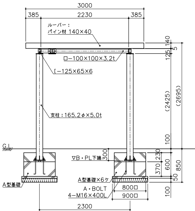
側面図 S＝ 1：40
