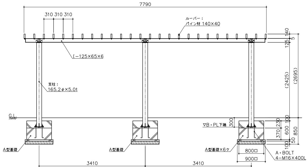
立面図 S＝ 1：40
