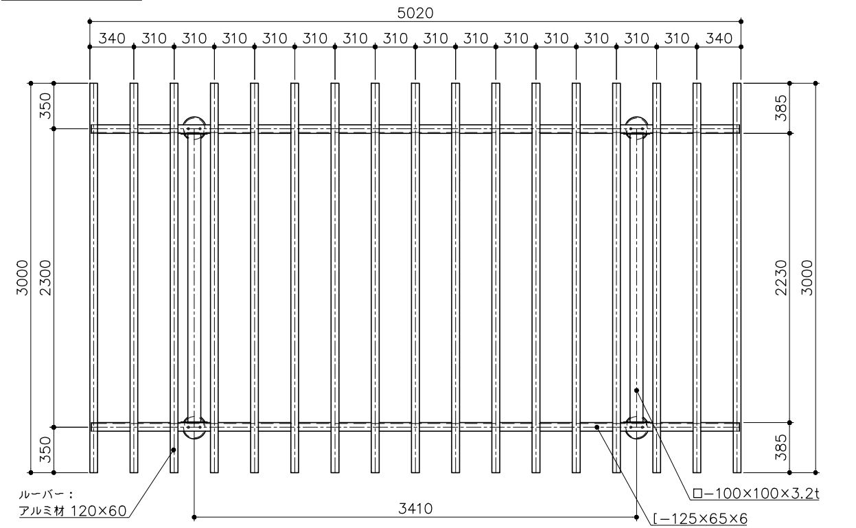
立面図 S= 1：30
