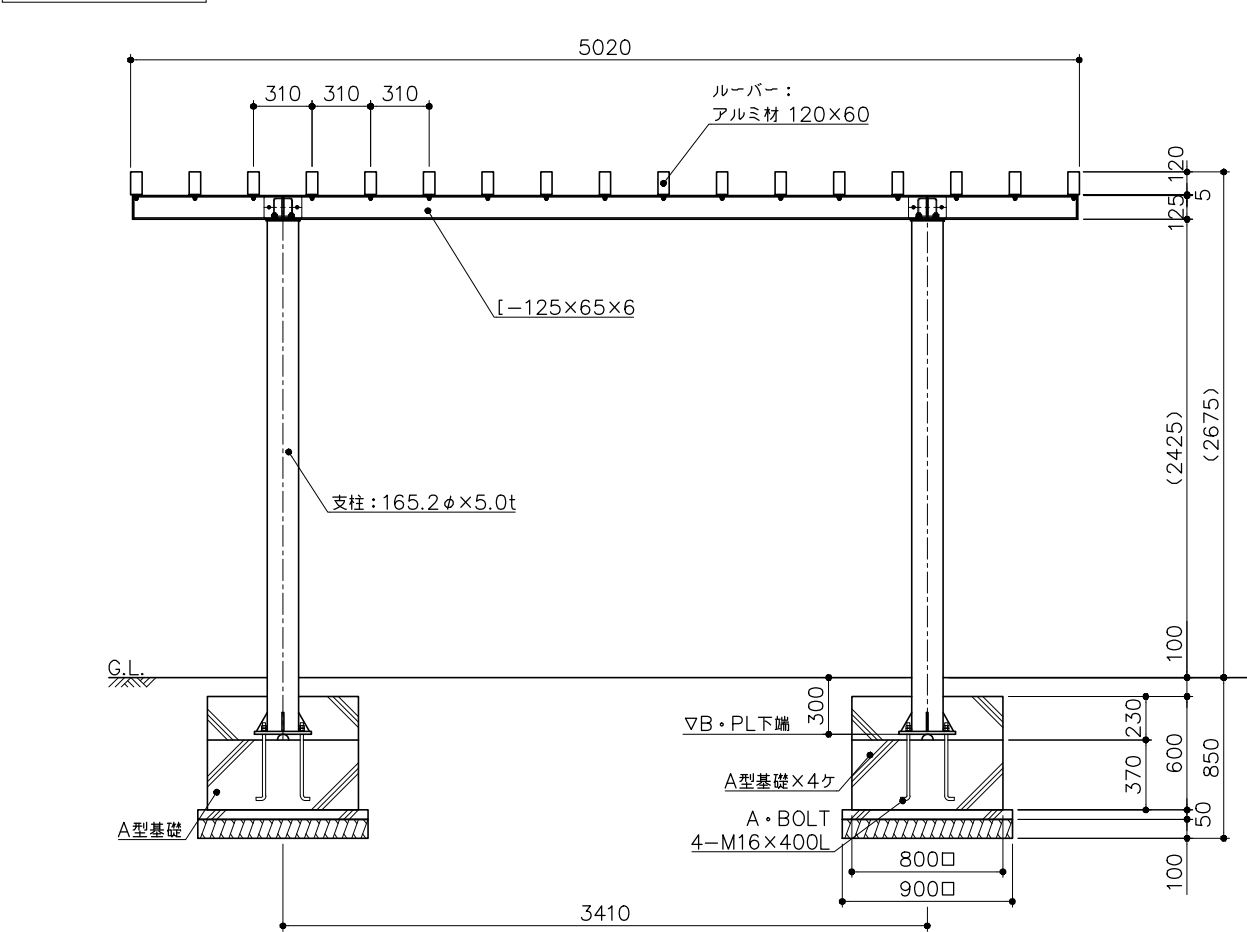
立面図 S= 1：30
