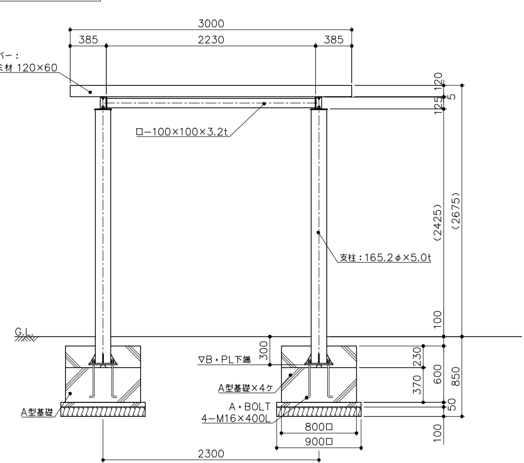
側面図 S= 1：30
