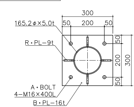
アンカープラン S= 1：10
