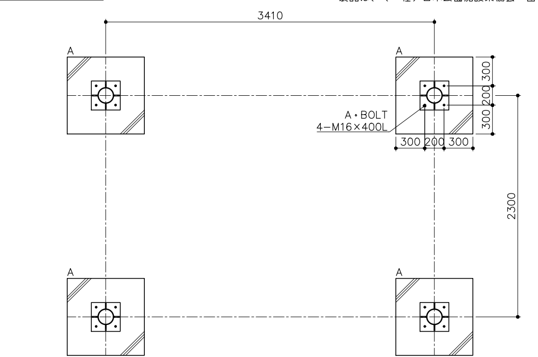
基礎平面図 S= 1：30
