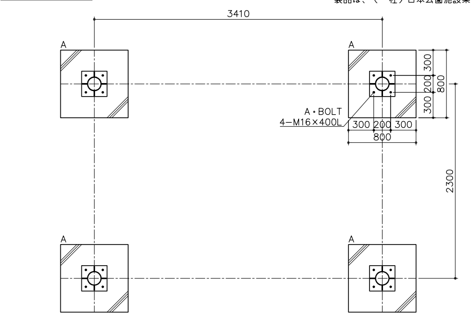
基礎平面図 S= 1 : 30
