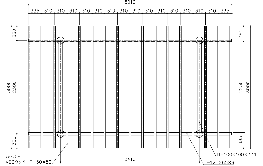
立面図 S= 1 : 30
