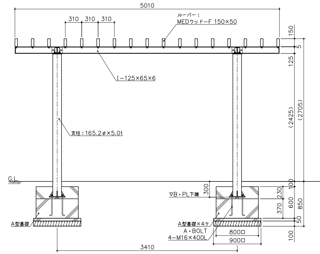
立面図 S= 1 : 30
