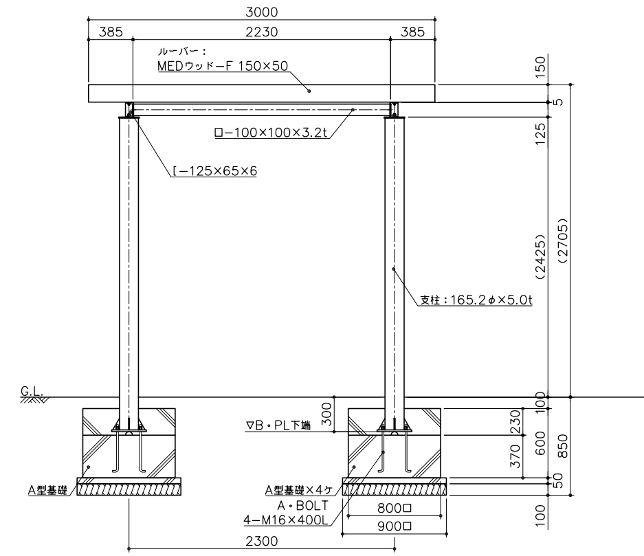
側面図 S= 1 : 30
