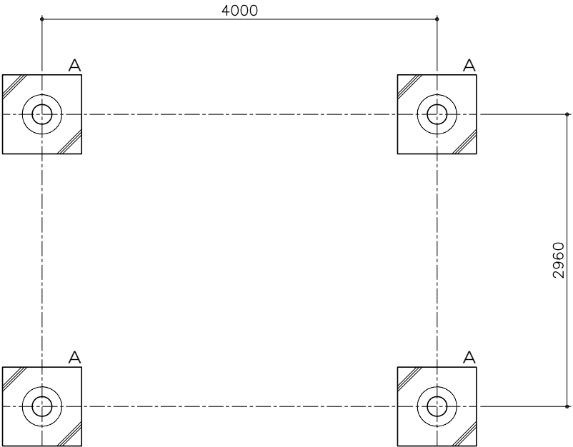
基礎平面図 S= 1：40
