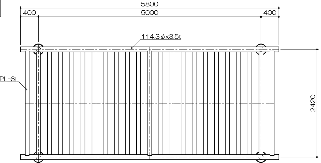
平面図 S= 1 : 50
