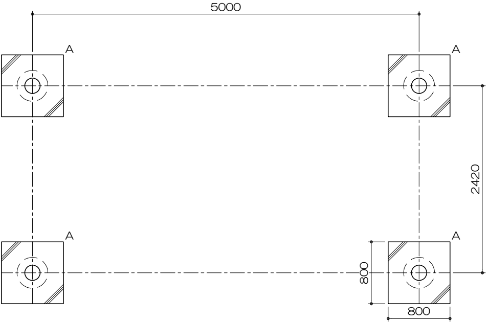
基礎平面図 S= 1 : 50
