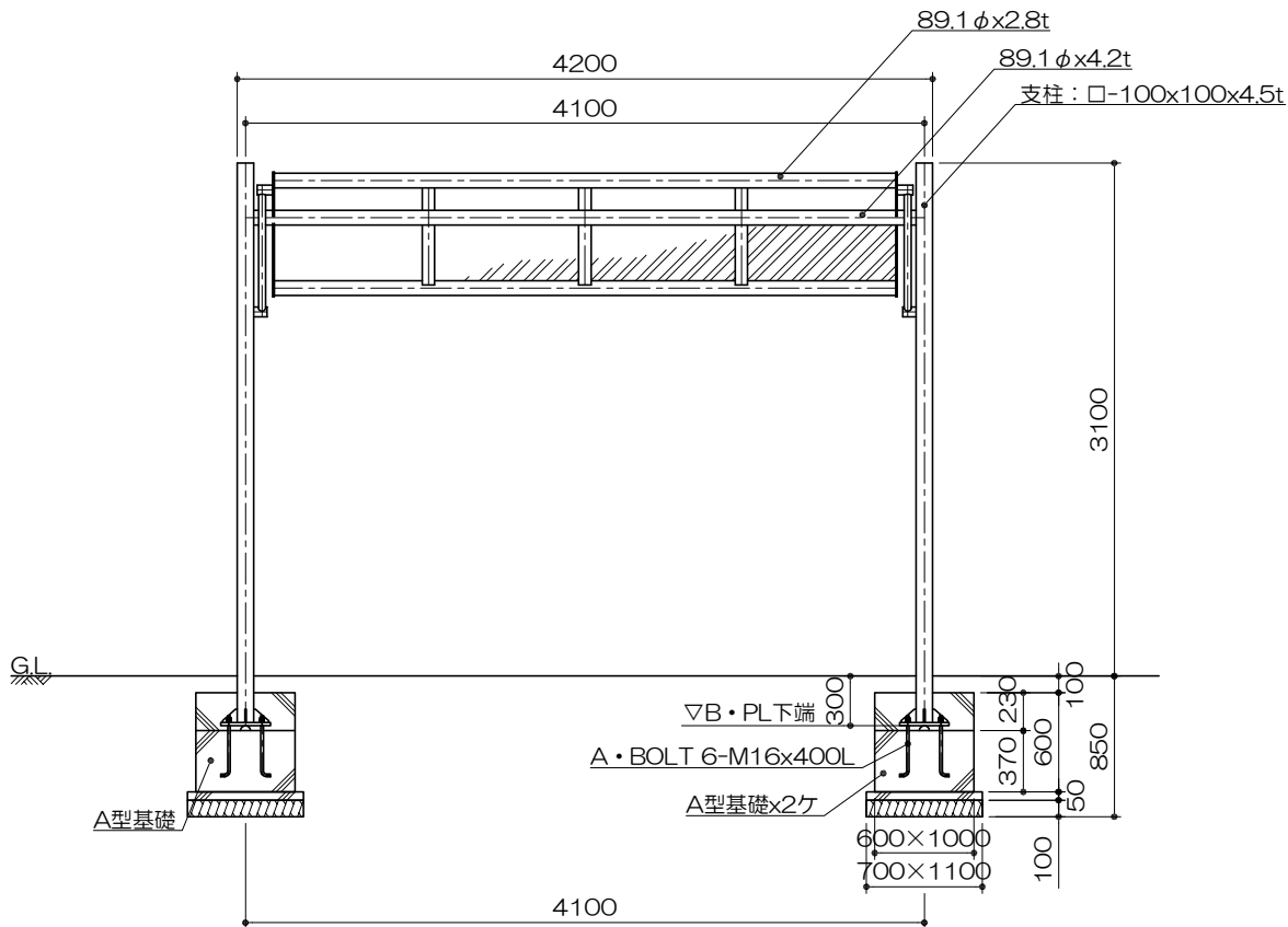
立面図 S= 1 : 50
