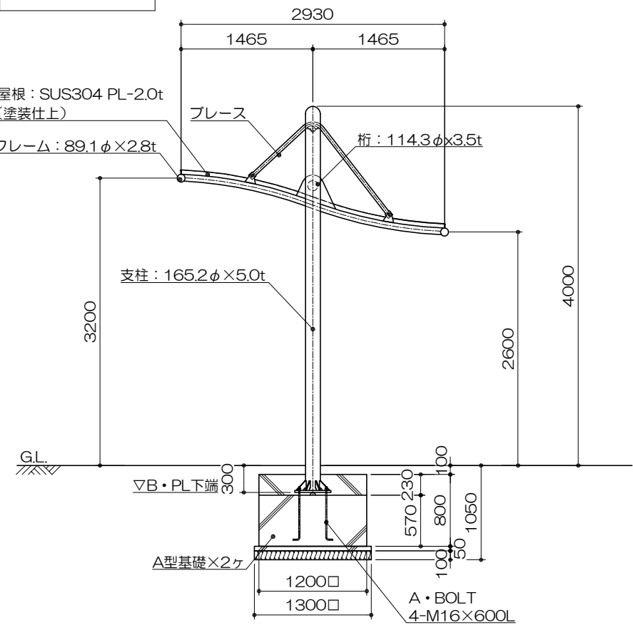
側面図 S= 1 : 60
