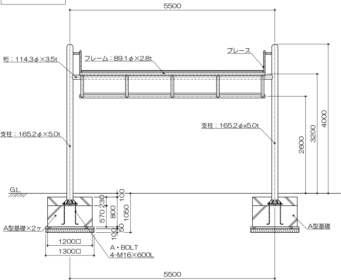
立面図 S= 1 : 60
