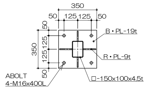
アンカープラン S= 1 : 20
