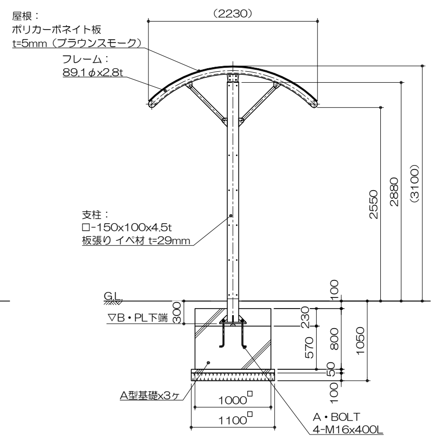
側面図 S= 1 : 50
