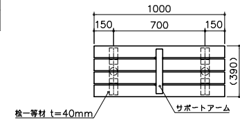
ベンチ (L=1000) 平面図 S= 1:20
