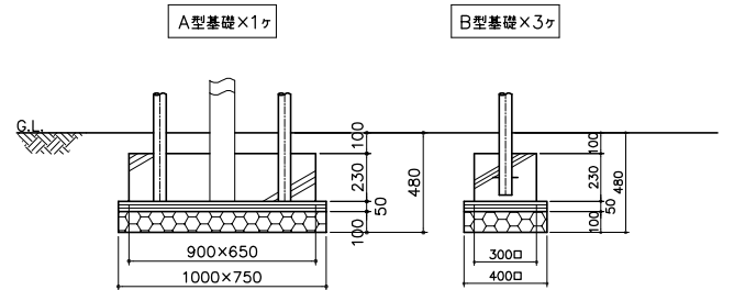
基礎リスト S= 1:20
