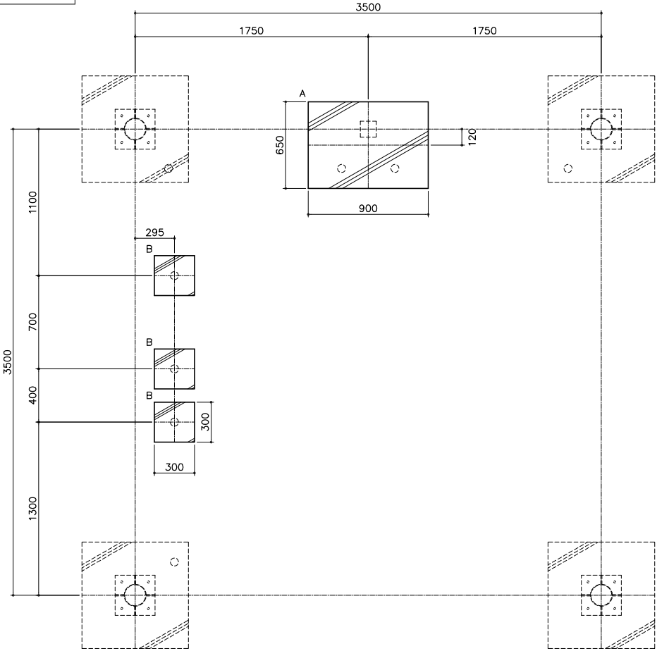
基礎平面図 S= 1:20
