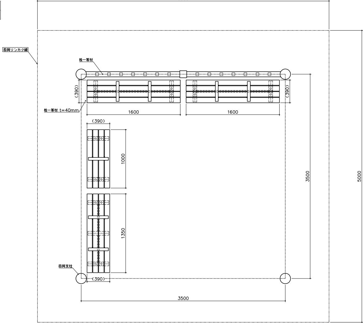
平面図 S= 1:20
