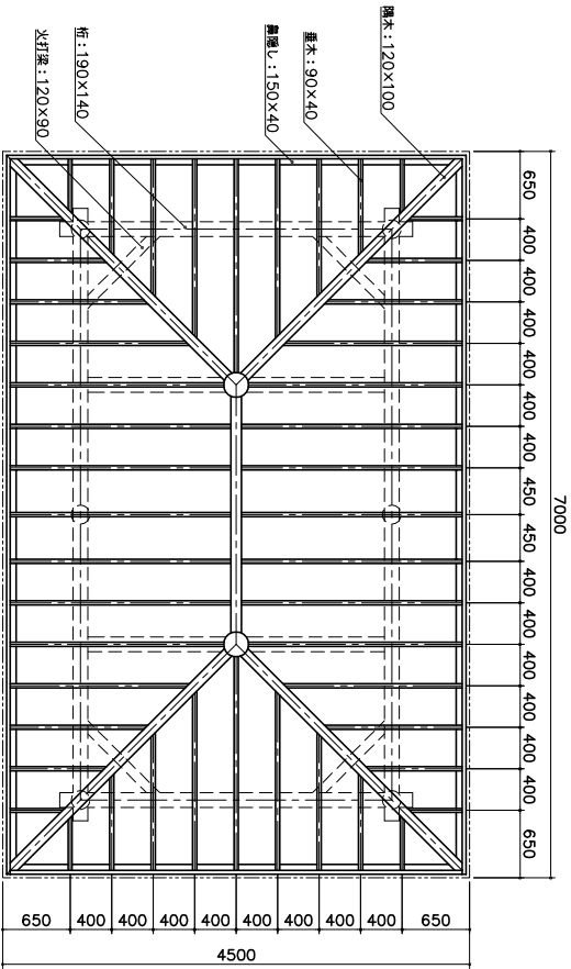
小屋伏図 S=1:40
