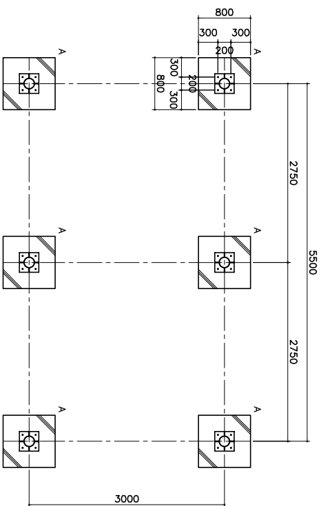
基礎平面図 S=1:40
