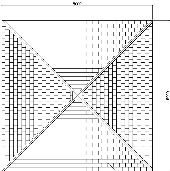
屋根伏図 S= 1:30
