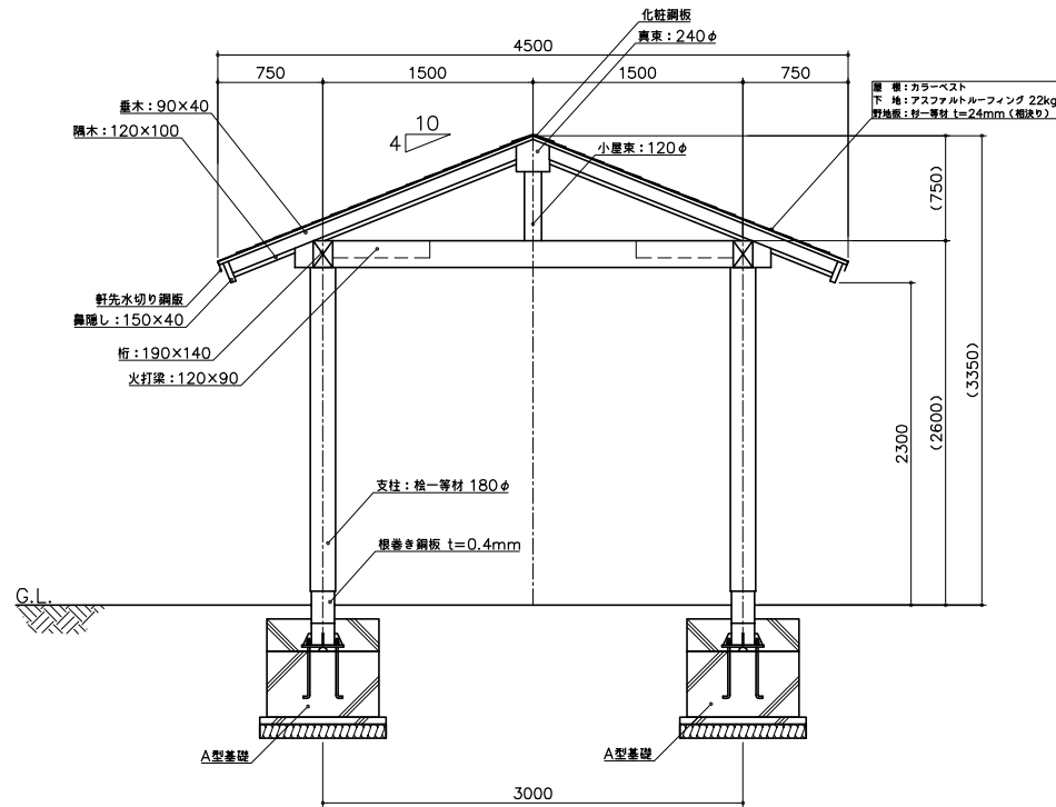
矩計図 S= 1:30
