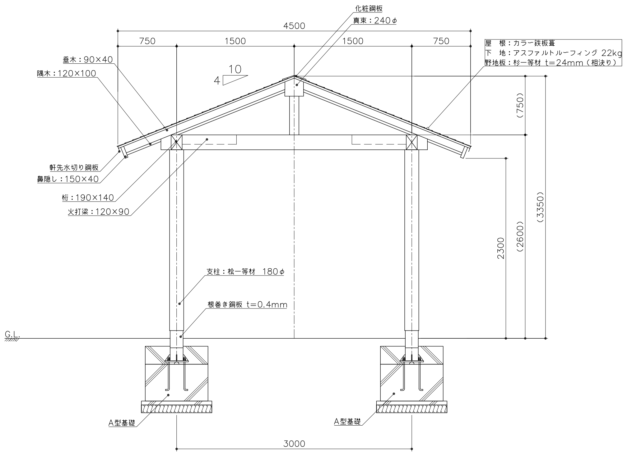
矩計図 S= 1:30
