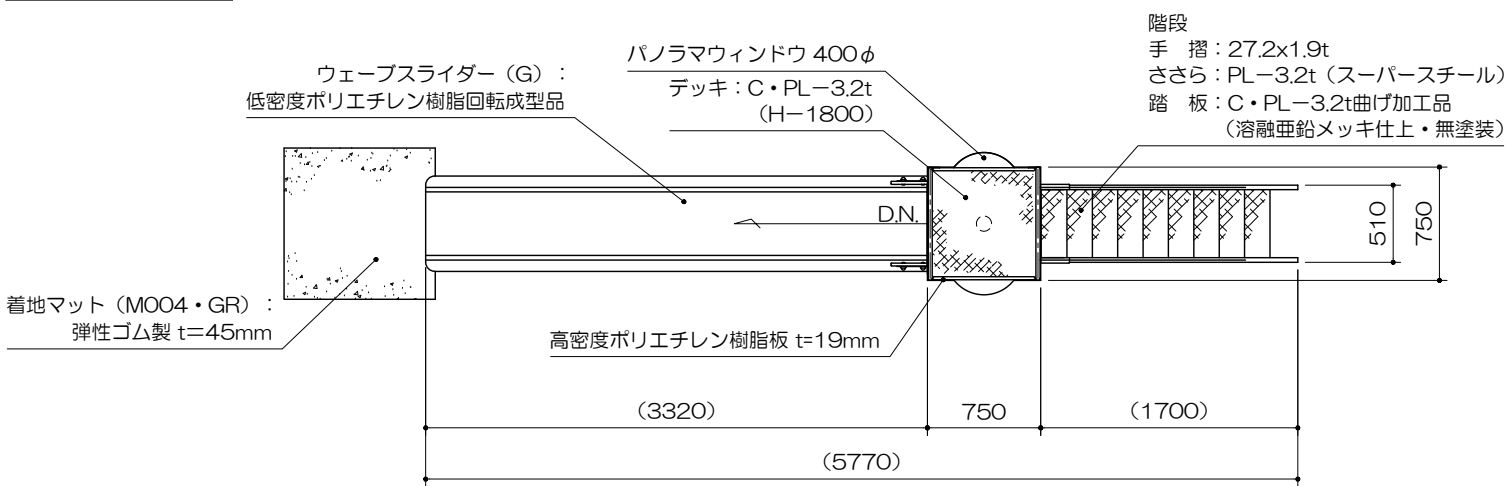
平面図 S= 1 : 50
