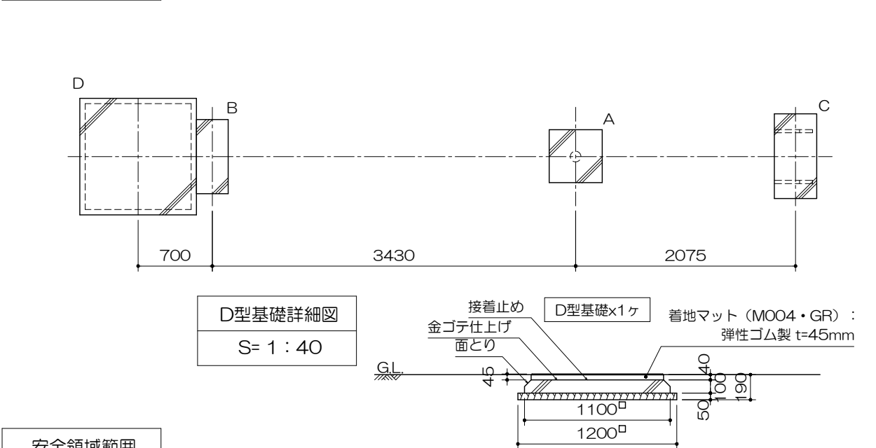
基礎平面図 S= 1 : 50
