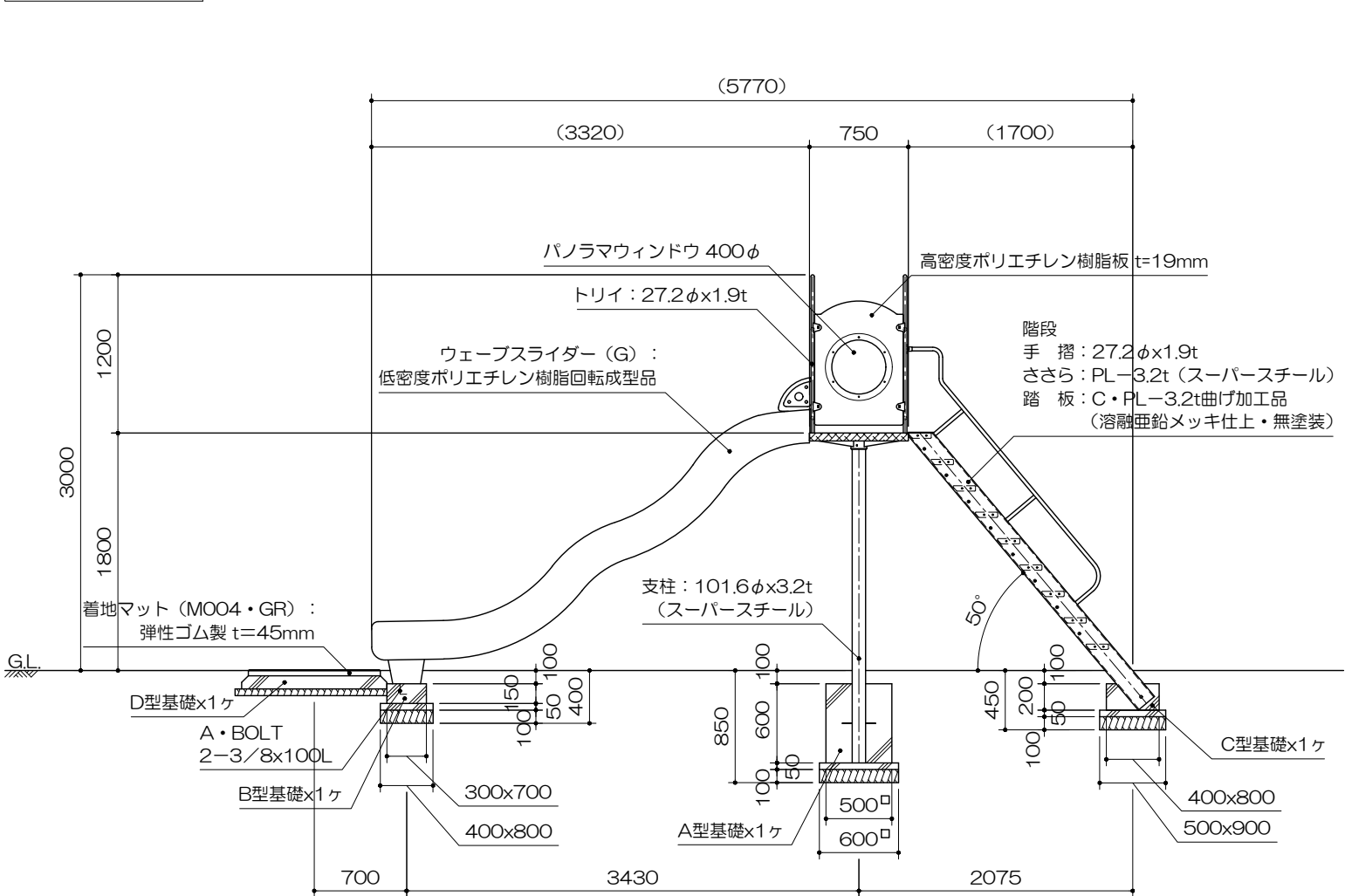
立面図 S= 1 : 50
