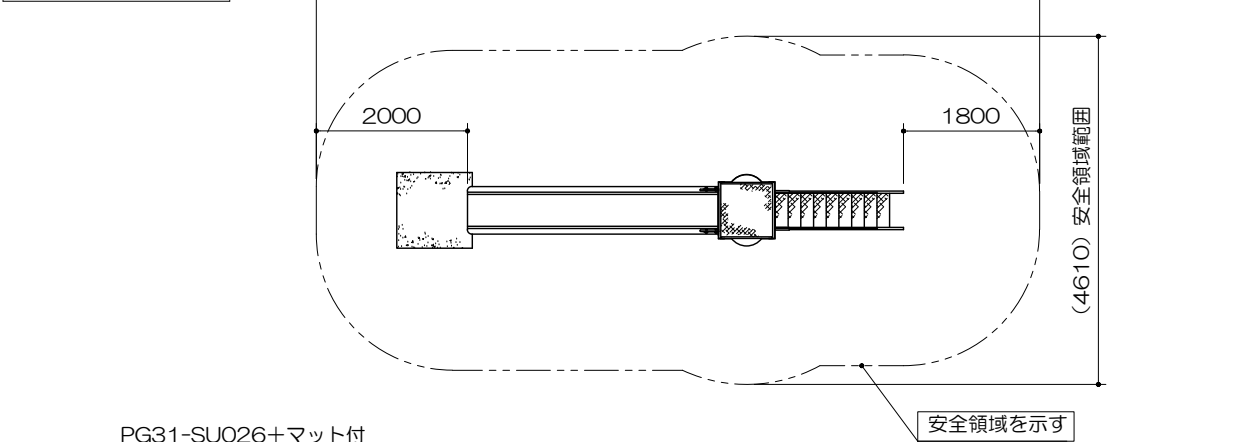
安全領域範囲 S= 1 : 100
